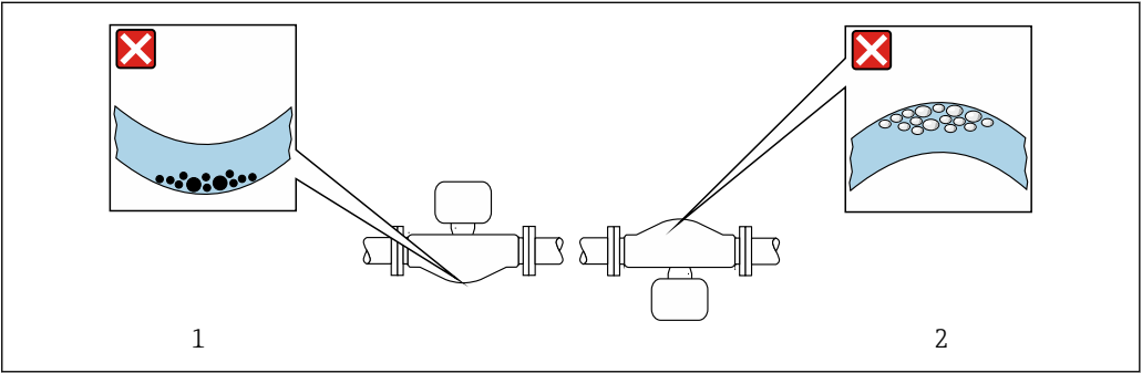
☒ 24 弓形計測チューブセンサの取付方向
