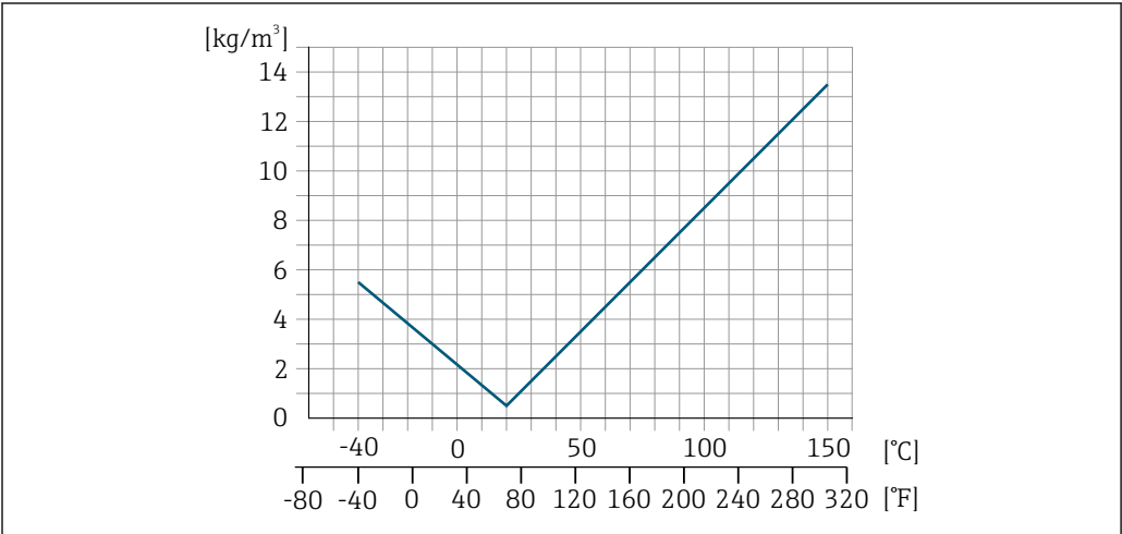
図 22 現場密度調整、例：+20 °C (+68 °F) 時
