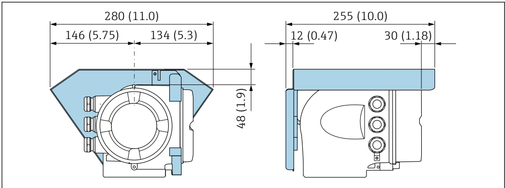
38 単位 mm (in)
