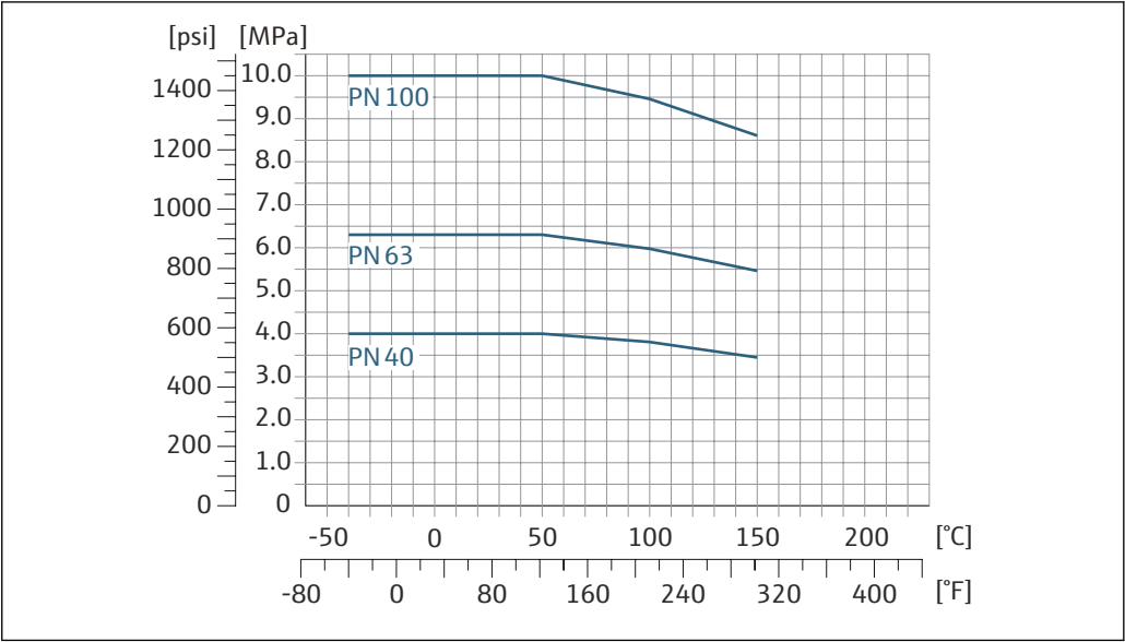
27 フランジ材質 1.4404 (SUS F316 または F316L 相当)
