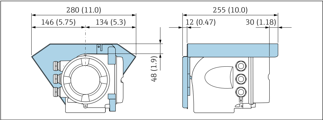
25 単位 mm (in)
