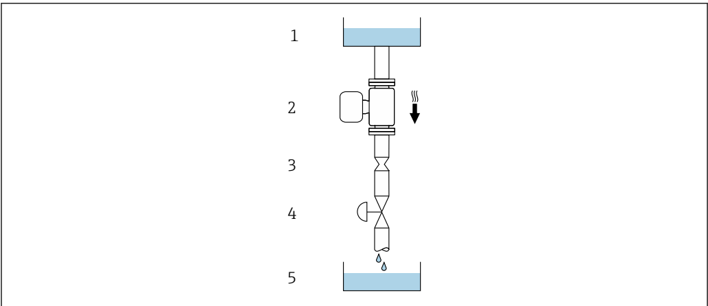
図 23 下向き配管への設置（例：バッチアプリケーション用）
