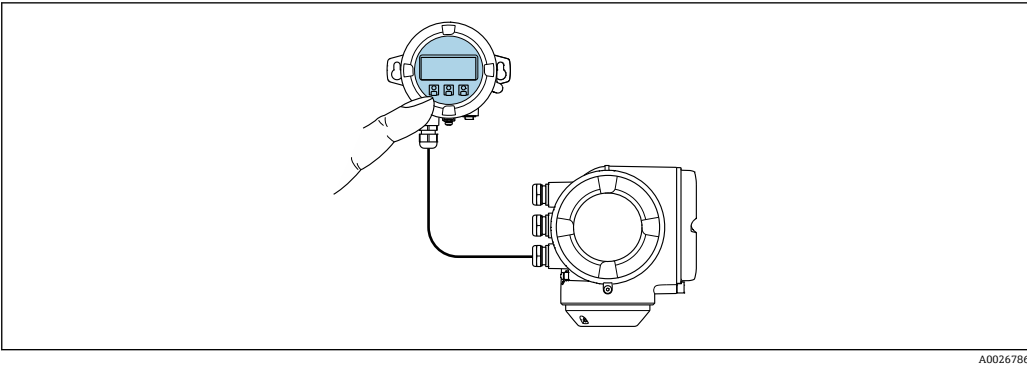
図 48 分離型ディスプレイと操作モジュール DKX001 を介した操作
