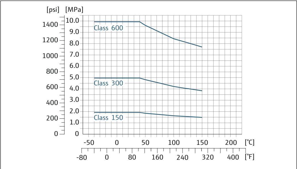
28 フランジ材質 1.4404 (SUS F316 または F316L 相当)
