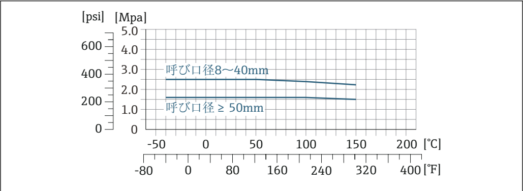
図 30 フランジ材質 1.4404 (SUS 316 または 316L 相当)
