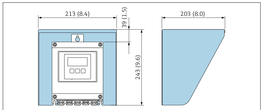
29 Proline 500 – デジタル用の日除けカバー、単位 mm (in)
