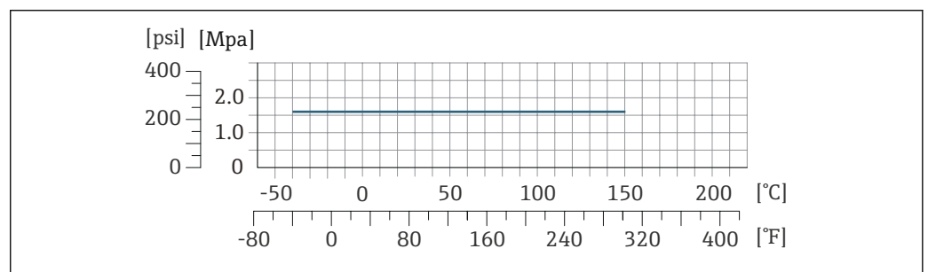
図 39 接続部の材質 1.4404 (SUS 316 または 316L 相当)
