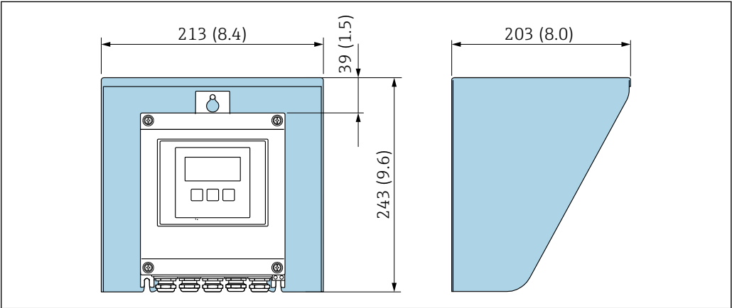
43 Proline 500 – デジタル用の日除けカバー、単位 mm (in)
