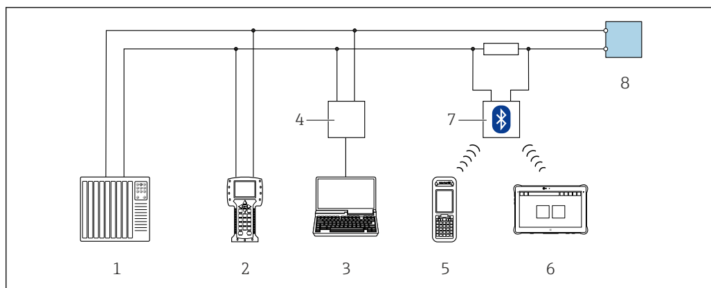
図 57 HART プロトコル経由のリモート操作用オプション（アクティブ）
