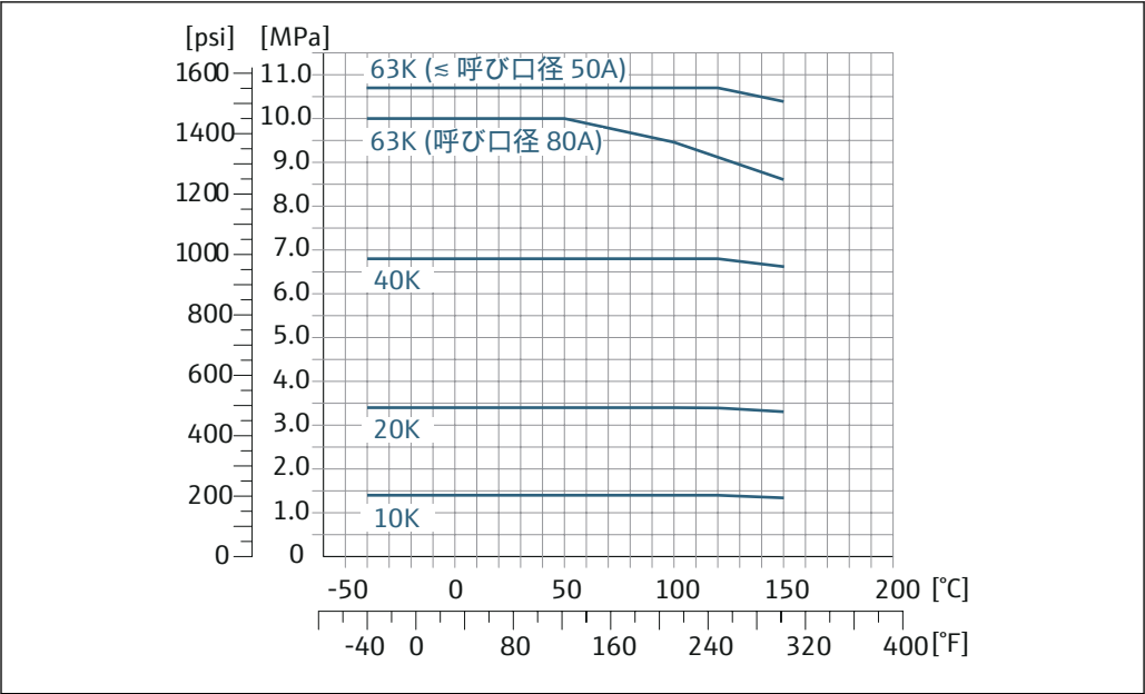
図 34 フランジ材質 1.4404 (SUS F316 または F316L 相当)
