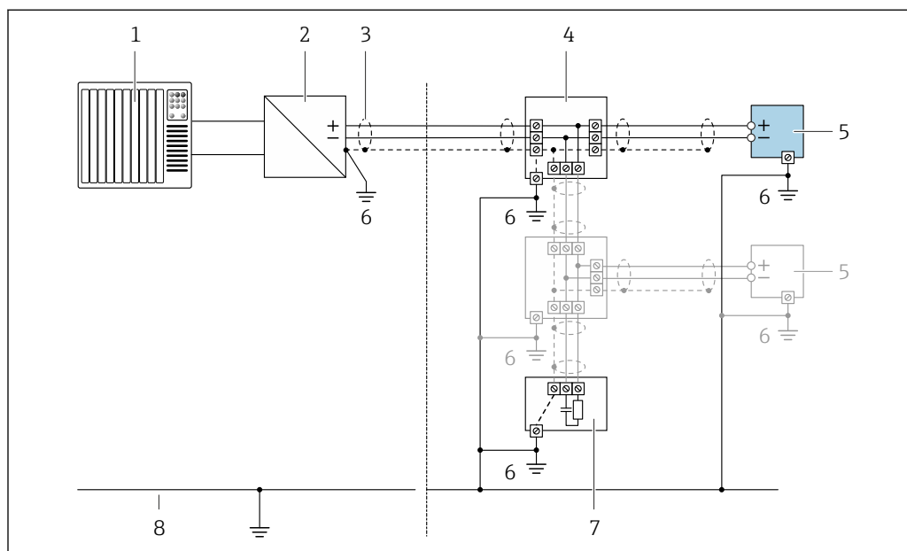
5 PROFIBUS PA の接続例
