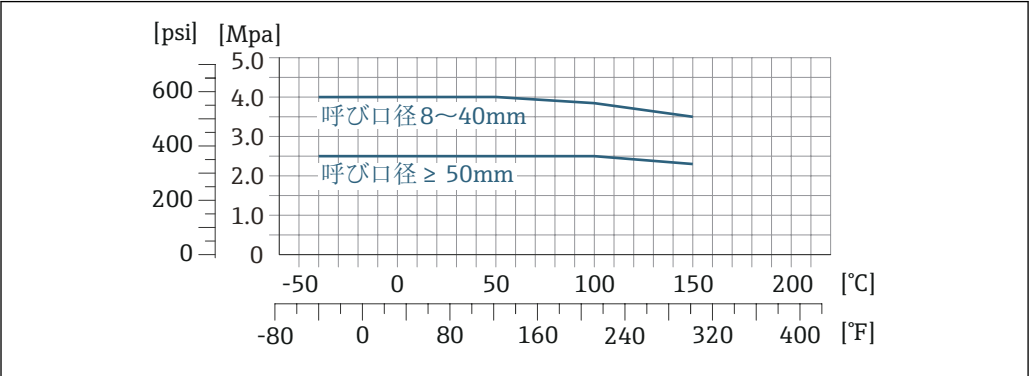
図 36 接続部の材質 1.4404 (SUS 316 または 316L 相当)
