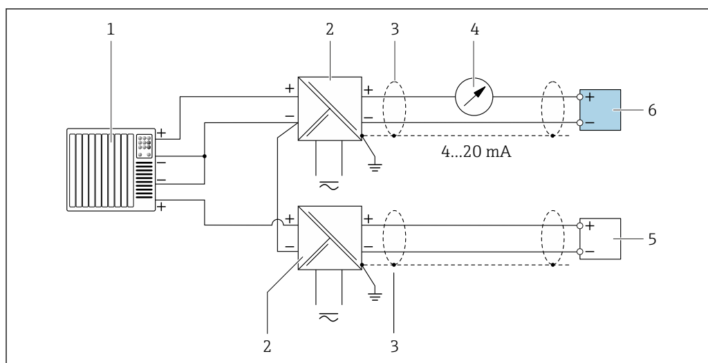
4 マイナスコモン の HART 入力 (パッシブ) の接続例
