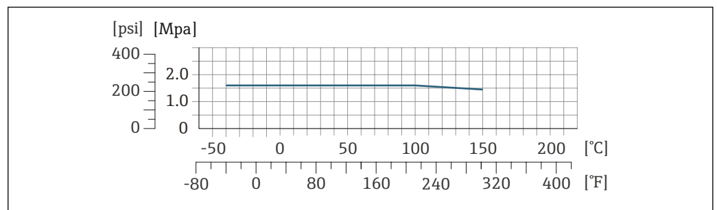
図 38 接続部の材質 1.4404 (SUS 316 または 316L 相当)
