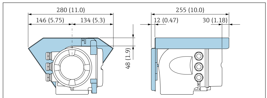
30 Proline 500 用の日除けカバー、単位 mm (in)
