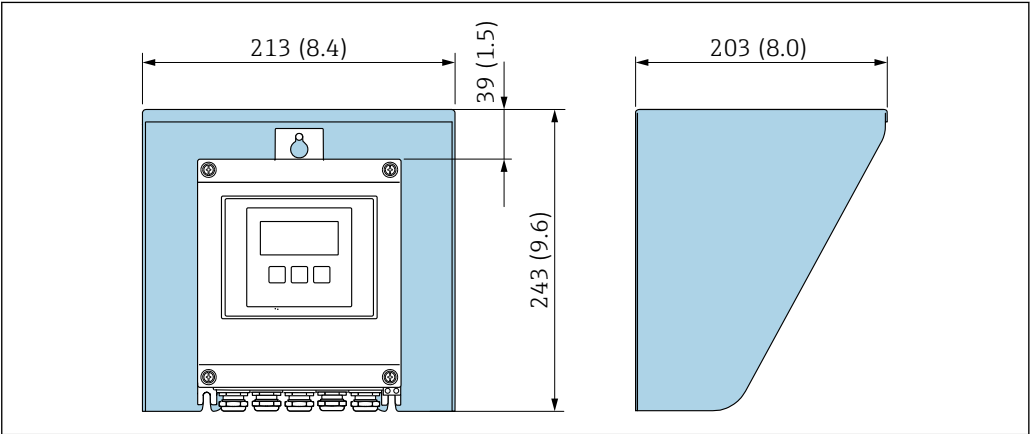
49 Proline 500 – デジタル用の日除けカバー、単位 mm (in)
