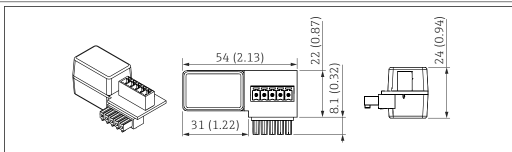
6 Dimensioni del resistore di comunicazione HART. Unità di misura mm (in)
