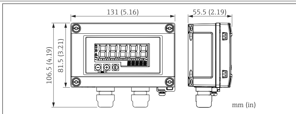
5 Dimensioni di RIA15 in custodia da campo. Unità di misura mm (in)
