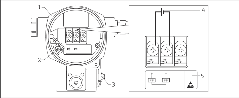
图 1 FOUNDATION Fieldbus 型仪表电气连接示意图
