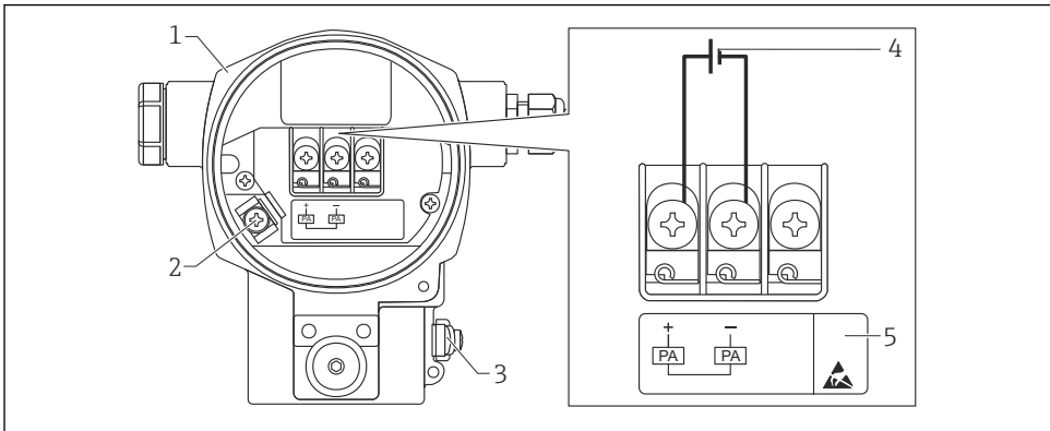
图 1 PROFIBUS® PA 电气连接示意图
