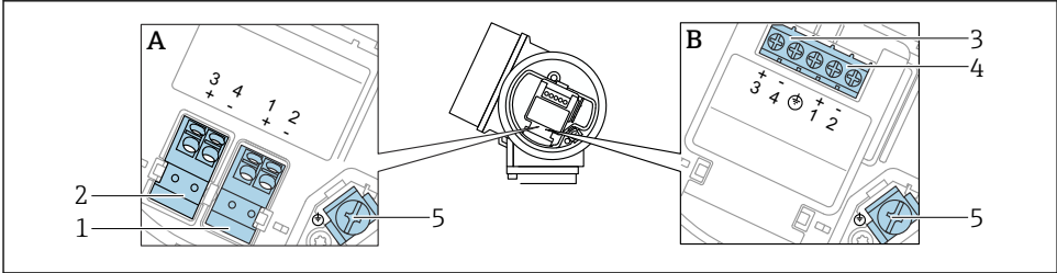
图 4 接线端子分配，两线制：4 ... 20 mA HART，开关量输出
