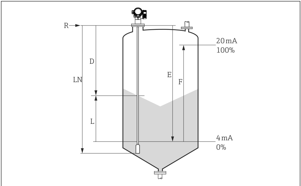
图 19 固体散料料位测量设置参数
