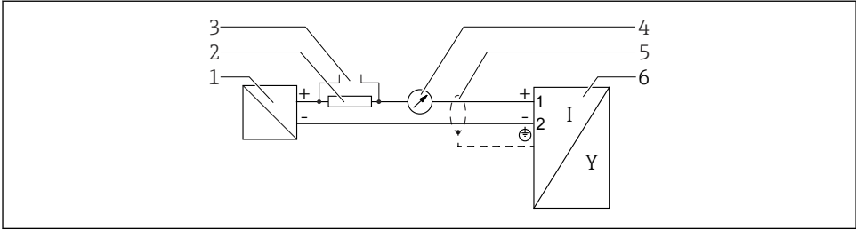
图 3 接线图：两线制：4 ... 20 mA HART
