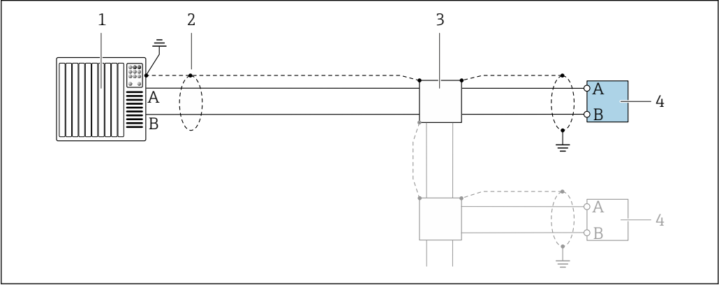
12 接线实例：Modbus RS485，非危险区和防爆 2 区；CI. I, Div. 2 防爆场合
