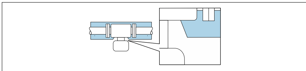
图 38 保温层延长颈裸露
