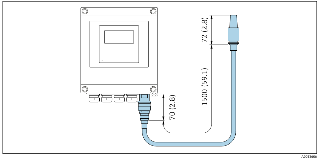
图 43 单位: mm (in)
