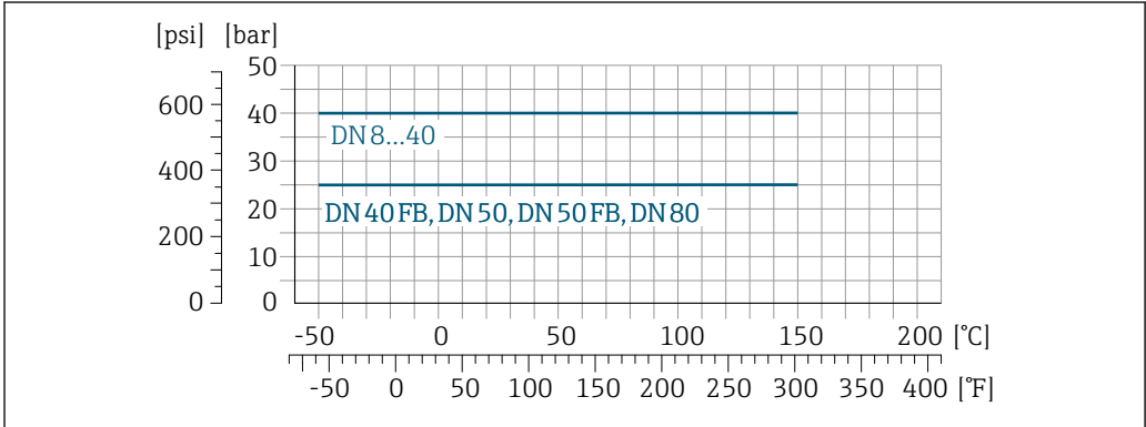
图 34 连接部件材质: 二级钛材
