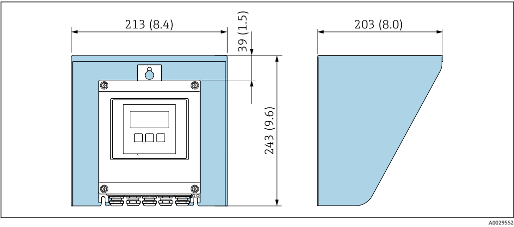
图 27 Proline 500（数字）变送器的防护罩的外形尺寸图；单位：mm (in)
