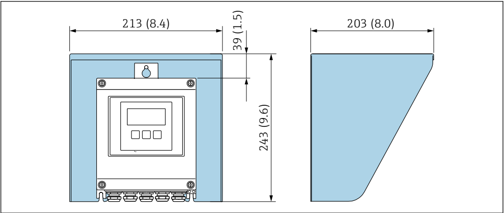
46 Proline 500 (数字) 变送器的防护罩的外形尺寸图; 单位: mm (in)
