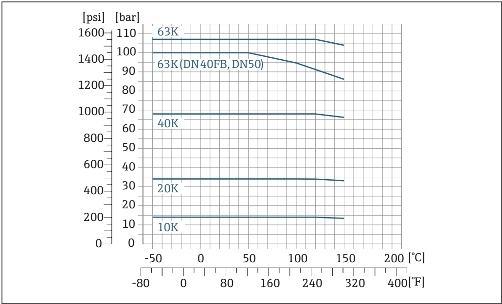
图 32 法兰材质: 1.4301 (304) ; 接液部件材质: 钛
