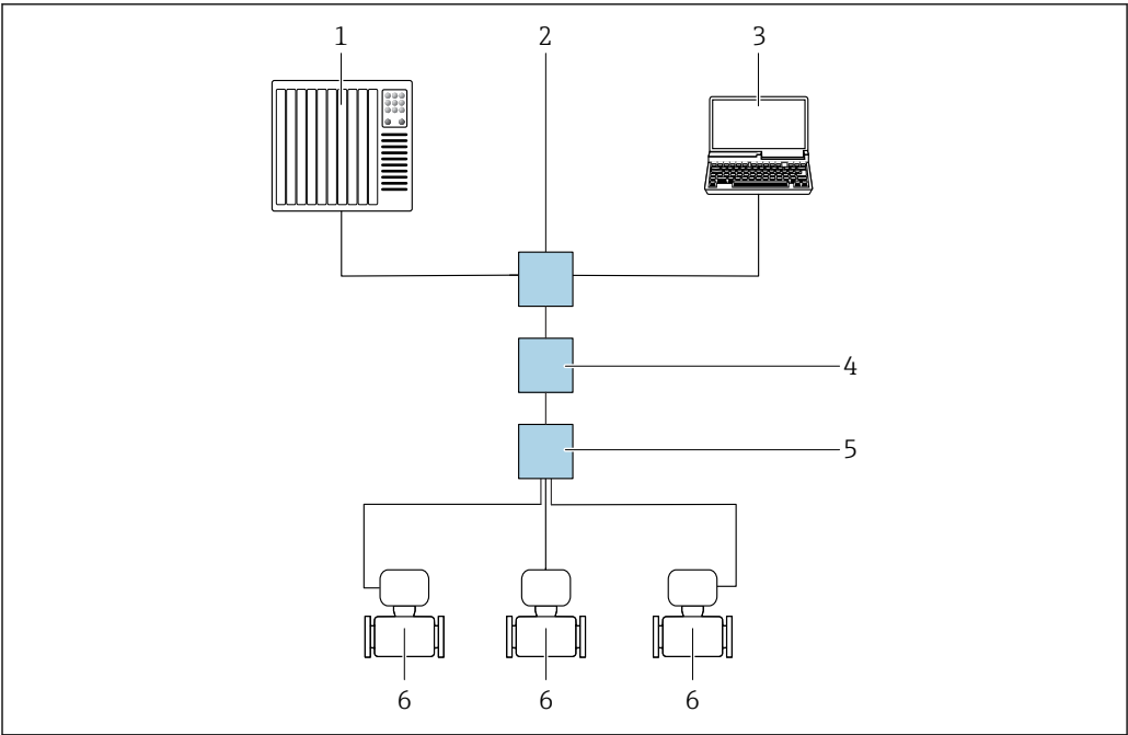
图 64 通过 APL 网络进行远程操作
