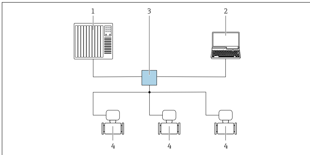
图 62 通过 PROFINET 网络进行远程操作：星形拓扑结构
