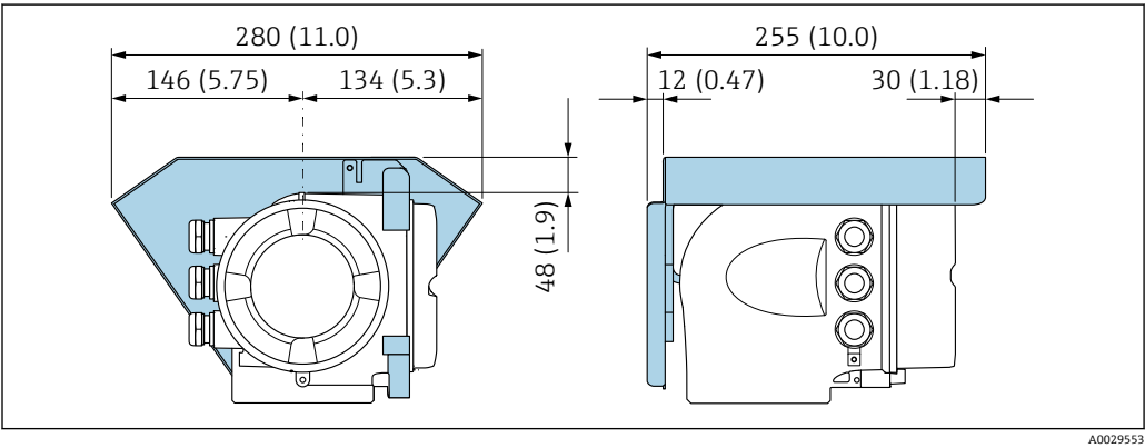
图 28 Proline 500（模拟）变送器的防护罩的外形尺寸图；单位：mm (in)
