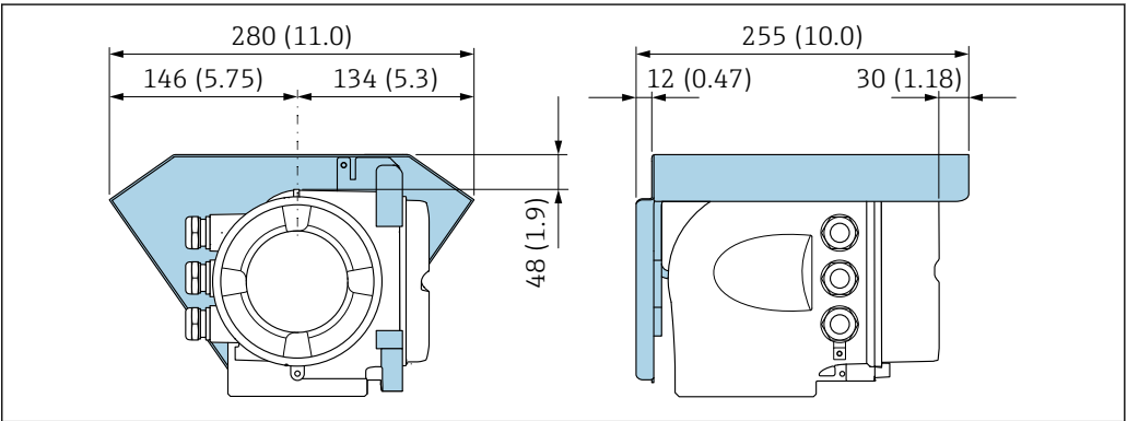
47 Proline 500 (模拟) 变送器的防护罩的外形尺寸图; 单位: mm (in)
