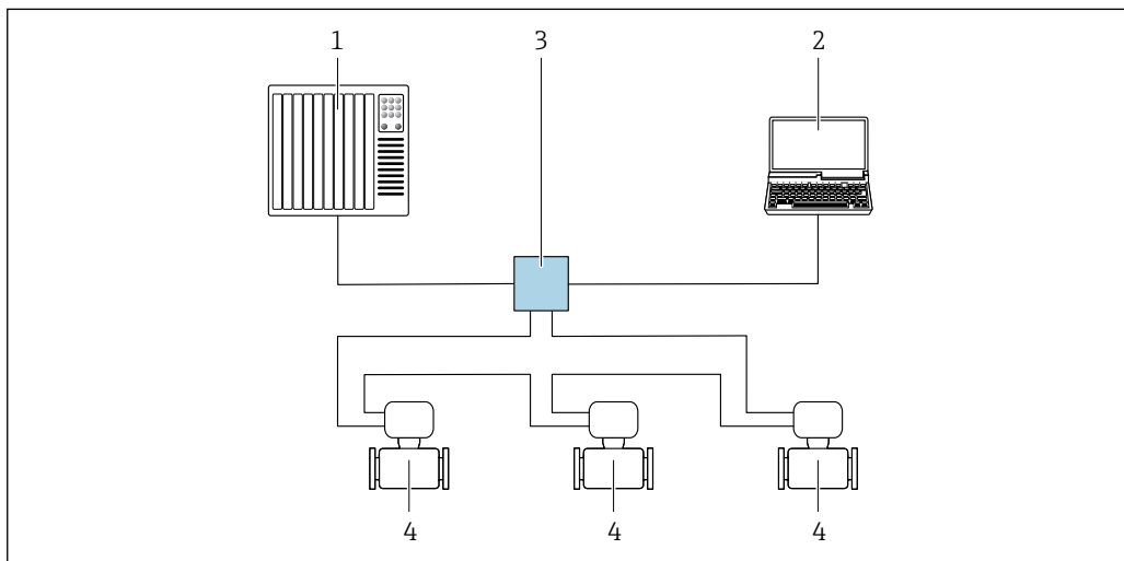
图 63 通过 PROFINET 网络进行远程操作：环形拓扑结构
