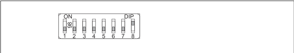
图 11 软件地址设定实例；开关 8 拨至“ON”位置；由操作菜单确定设备地址（Setup → Device address）。
