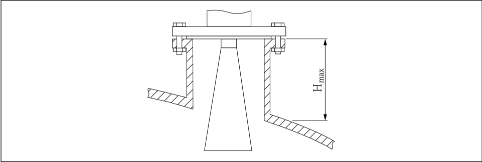
图 2 喇叭天线（FMR51）的安装短管高度示意图
