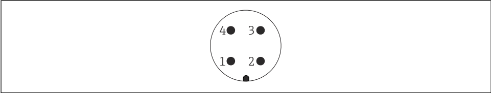
图 6 M12 插头的针脚分配
