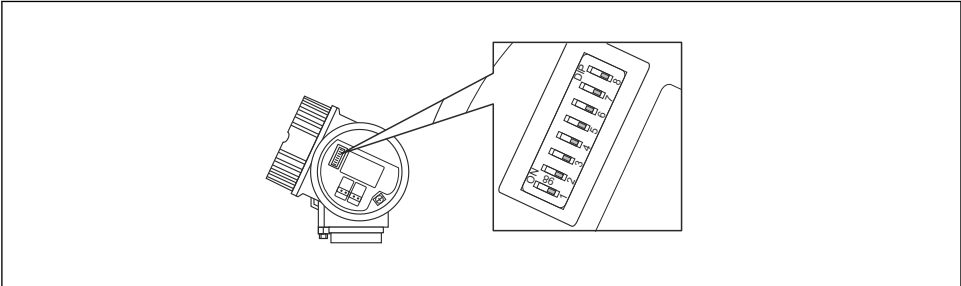
9 接线腔中的地址设定开关
