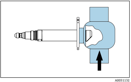
20 使用 Varivent 接头安装，带延长杆
