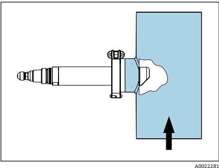
18 安装在 CUA262 流通式安装支架中
