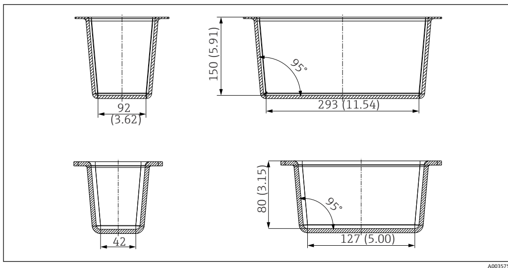
图 37 大型标定容器（上）和小型标定容器（下）；单位：mm (in)
