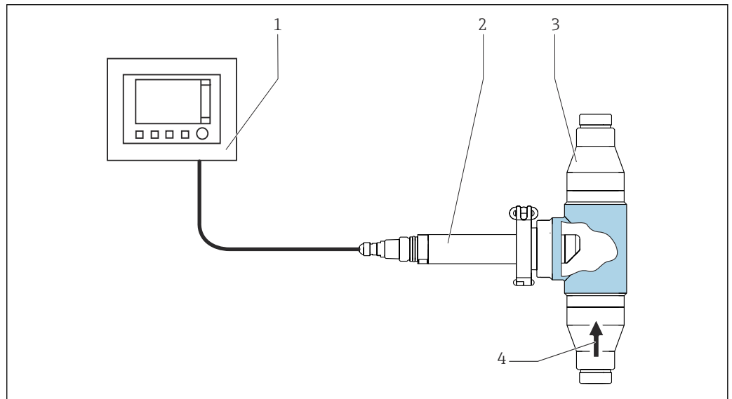
图 11 测量系统示例, 使用 CUA252 流通式安装支架, 针对不锈钢传感器
