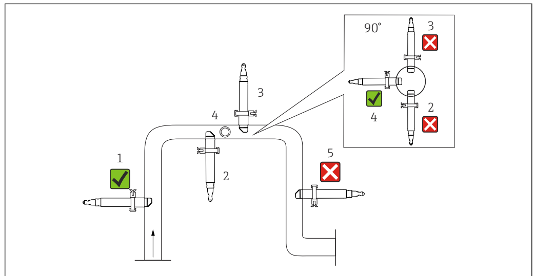
图 8 管道中允许和不可接受的方向
