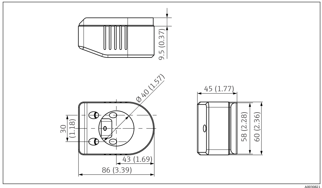
图 7 固态标定模块 Calkit CUS52D; 单位: mm (in)
