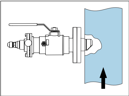
图 13 通过 CUA451 可伸缩式安装支架安装
