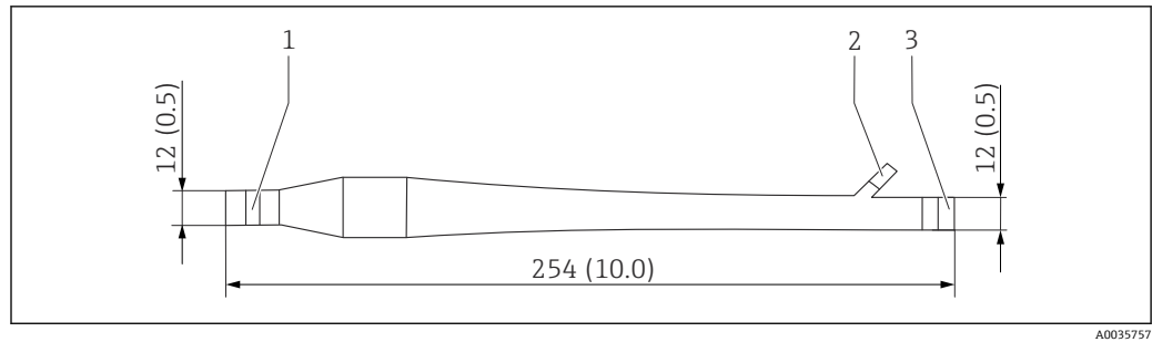
图 42 消泡装置示意图；单位：mm (in)
