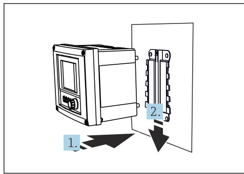
12 Gerät anhängen, einklicken
