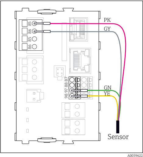
26 Sensoren mit zusätzlicher Versorgungsspannung
