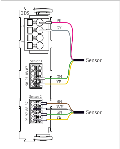
27 Sensoren mit und ohne zusätzliche Versorgungsspannung am Sensormodul 2DS
