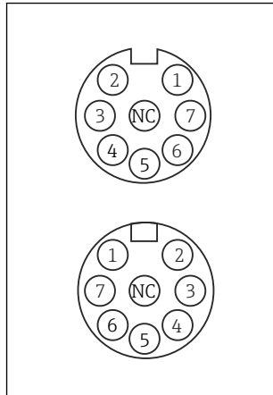
29 M12-Belegung Oben: Buchse Unten: Stecker (jeweils Draufsicht)
