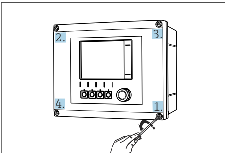
13 Gehäuseschrauben mit Kreuzschlitz-Schraubendreher kreuzweise lösen
