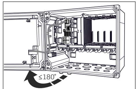
14 Displaydeckel öffnen, max. Öffnungswinkel 180° (abhängig von Einbausituation)
