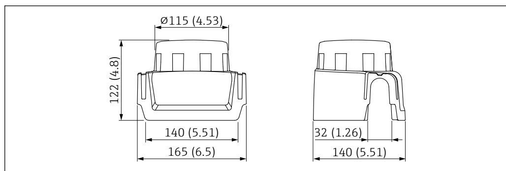
45 Защитный козырек для однокамерного корпуса, алюминий или 316L. Единица измерения мм (дюйм)
