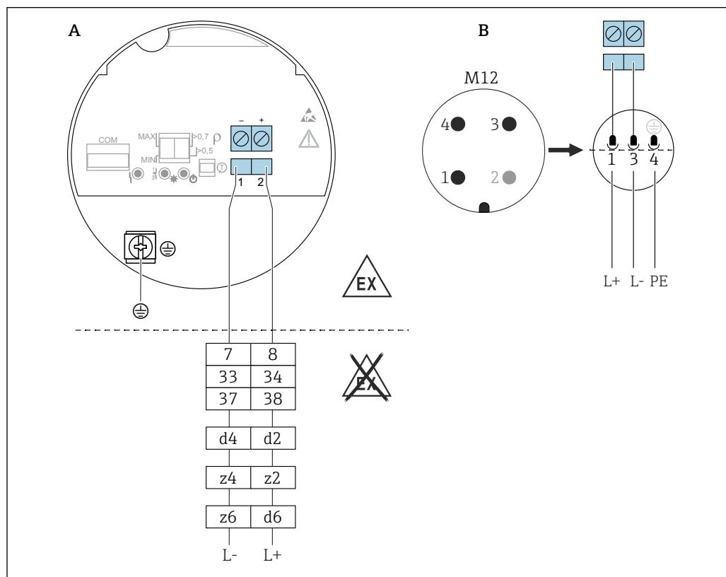
25 Выход ЧИМ, электронная вставка FEL67
