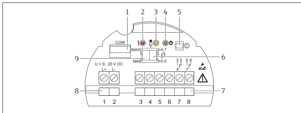
32 Пример: электронная вставка FEL64DC
