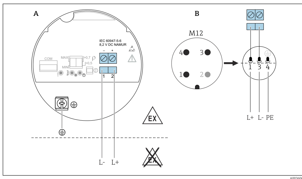
27 2-проводное подключение NAMUR \geq 2,2 \text{ мА} / \leq 1,0 \text{ мА} , электронная вставка FEL68
