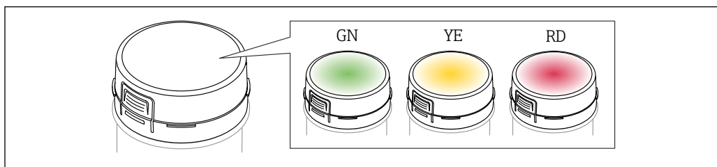
47 Светодиодный модуль содержит светодиоды, которые горят зеленым (GN), желтым (YE) или красным (RD) светом
