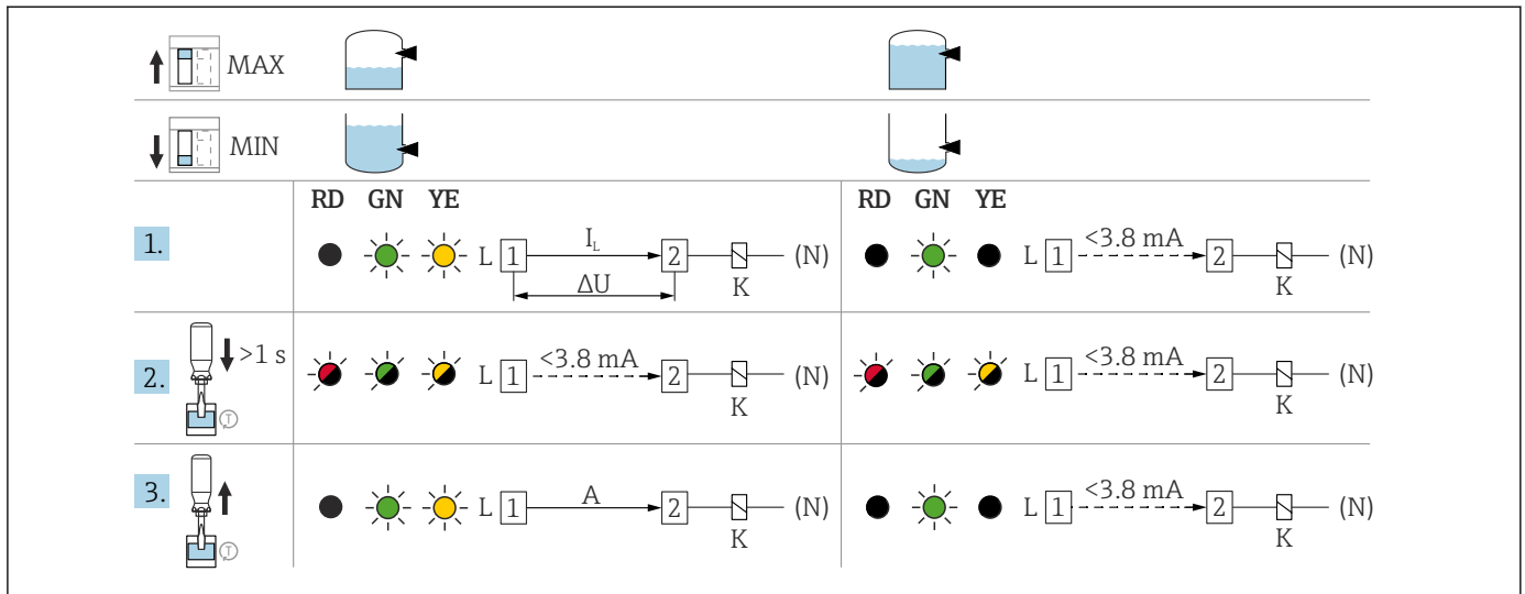
35 Поведение при переключении и сигнализация вставки FEL61
