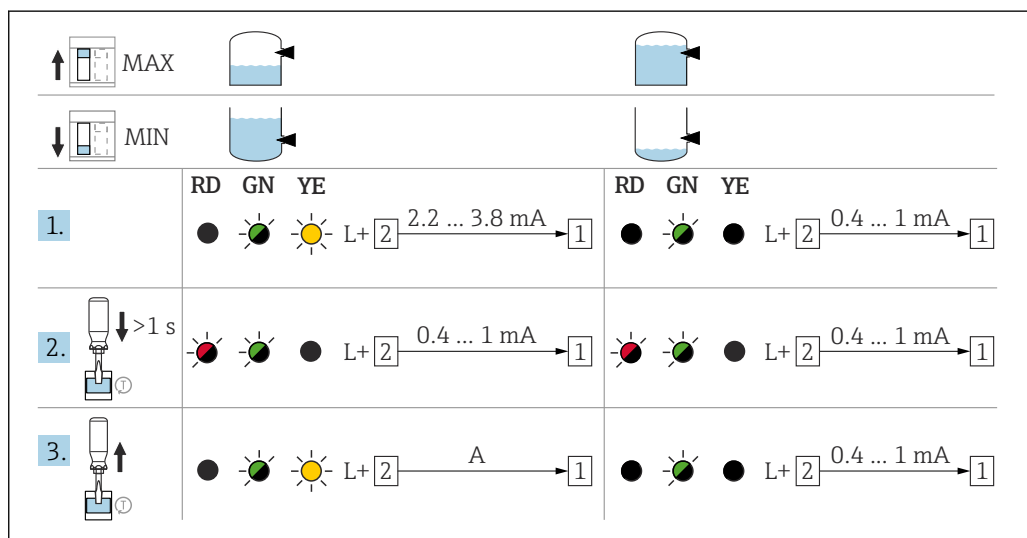
40 Поведение при переключении и сигнализация электроники NAMUR
