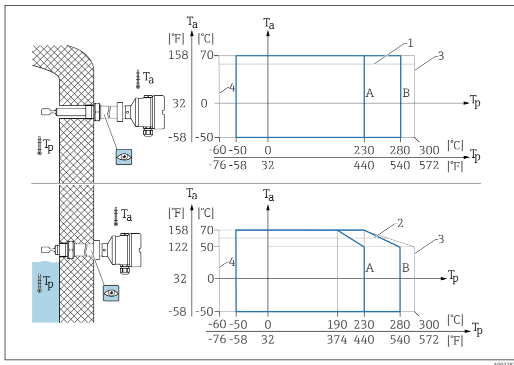
50 Зависимость допустимой температуры окружающей среды T_a в зоне корпуса от рабочей температуры T_p в резервуаре
