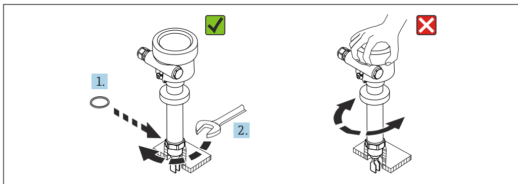
13 Прикручивание прибора
