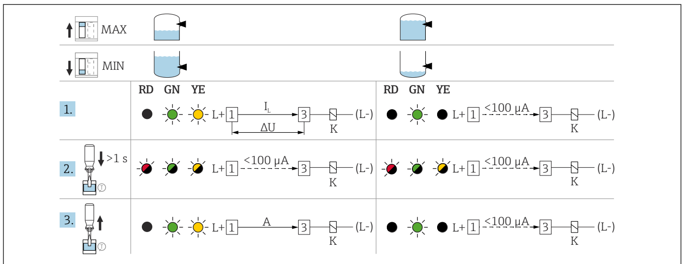
36 Поведение при переключении и сигнализация вставки FEL62
