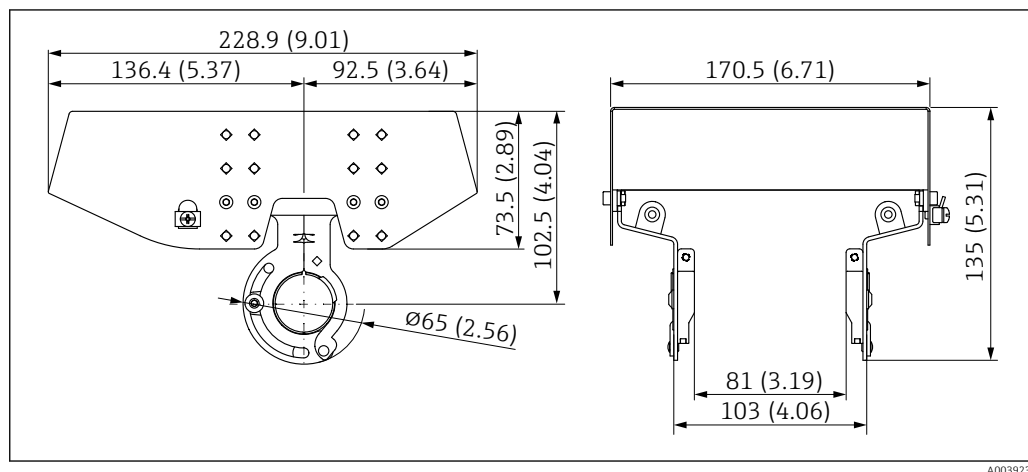
44 Защитный козырек для двухкамерного алюминиевого корпуса. Единица измерения мм (дюйм)
