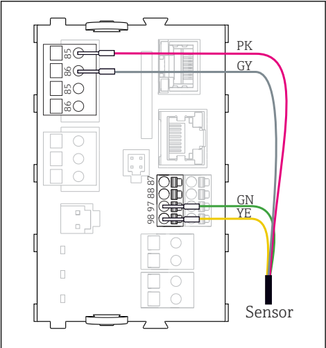
12 sensoren met extra voedingsspanning
