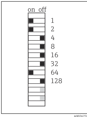
33 Geldig PROFIBUS adres 67
