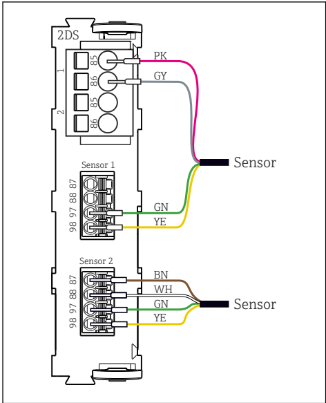
13 Sensoren met en zonder extra voedingsspanning op sensormodule 2DS
