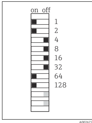
34 Geldig Modbus adres 195
