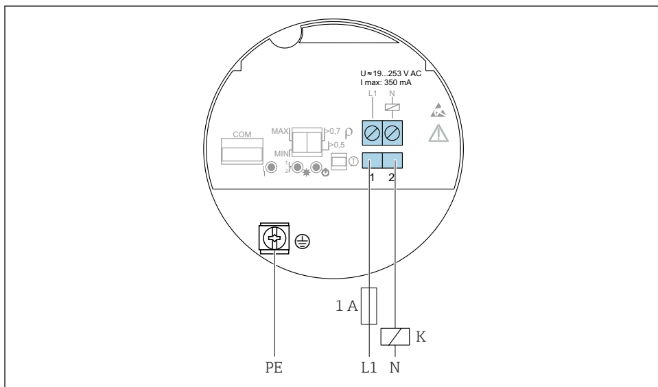
14 2-johtiminen vaihtovirta, elektroniikkakoke FEL61
