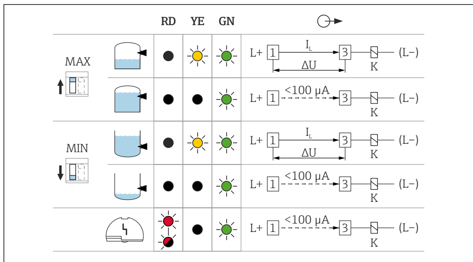
18 KytKentälähdön ja merkinannon toiminta, elektroniikkakoje FEL62
