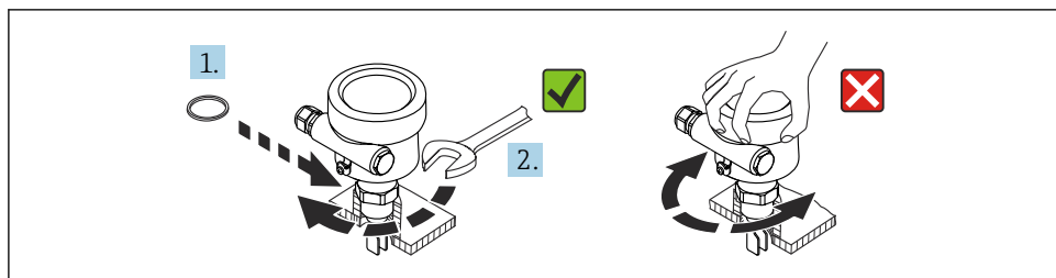
11 Laitteen ruuvaaminen
