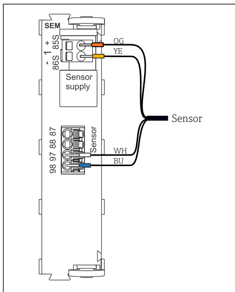
33 Připojení spektrometru k modulu SEM
