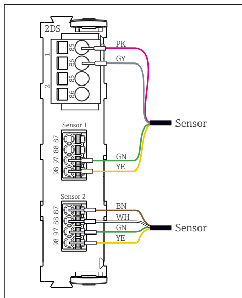
32 Senzory s přídavným napájením a bez něj na modulu senzorů 2DS
