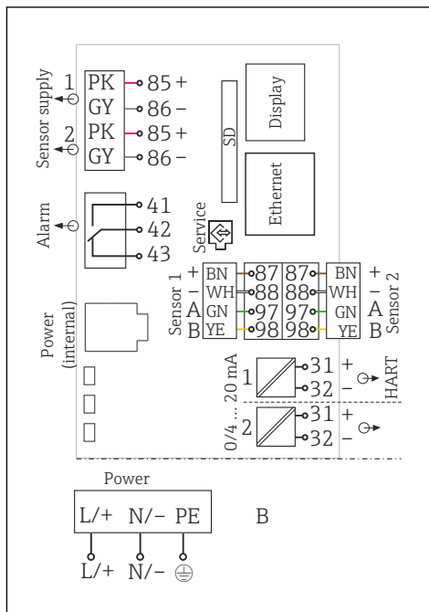
27 Kompletní schéma zapojení na příkladu BASE2-E a externího napájecího zdroje (B)
