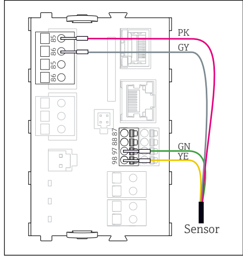
26 추가 공급 전압이 있는 센서
