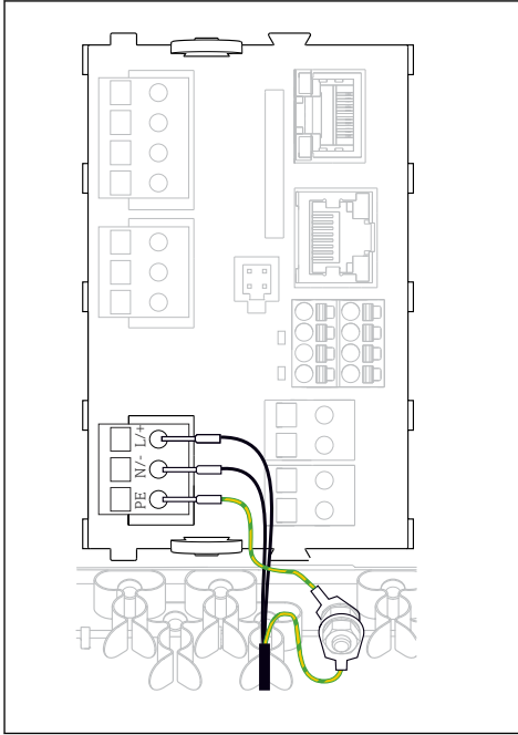
19 BASE2-H 또는 -L의 예를 사용한 전원 공급 장치 연결
