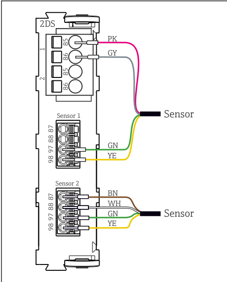
27 센서 모듈 2DS에서 추가 공급 전압이 있거나 없는 센서
