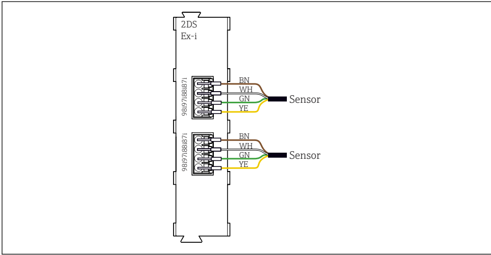
30 센서 통신 모듈 타입 2DS Ex-i에 추가 공급 전압이 없는 센서
