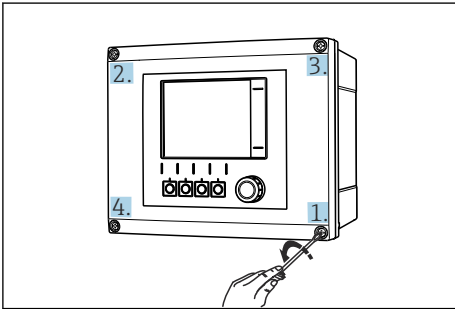
13 십자 드라이버를 사용해 하우징 나사를 대각선 순서로 풀기
