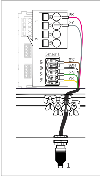
■ 28 M12 연결(예: 센서 모듈)
