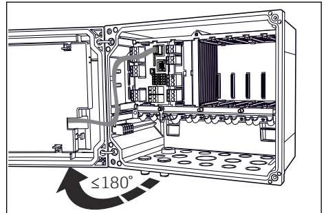
14 디스플레이 커버 열기, 최대 개방 각도 180°(설치 위치에 따라 다름)
