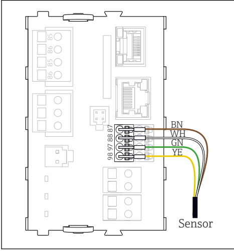
25 추가 공급 전압이 없는 센서
