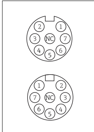
■ 29 M12 할당, 위: 소켓 아래: 커넥터(각각 평면도)
