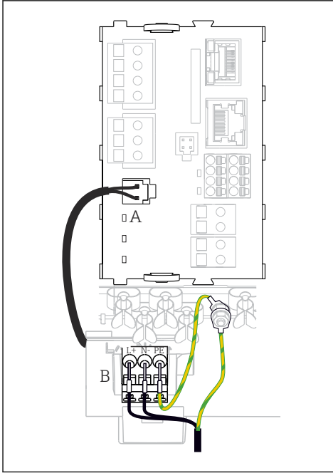
■ 22 BASE2-E의 예를 사용한 전원 공급 장치 연결
