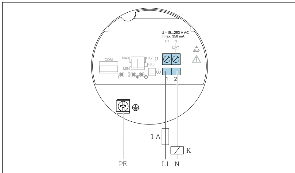
13 2-tråds AC, elektronikkinnsats FEL61
