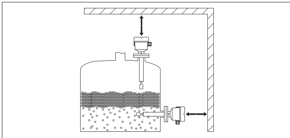
7 Ta hensyn til klaring på utsiden av tanken
