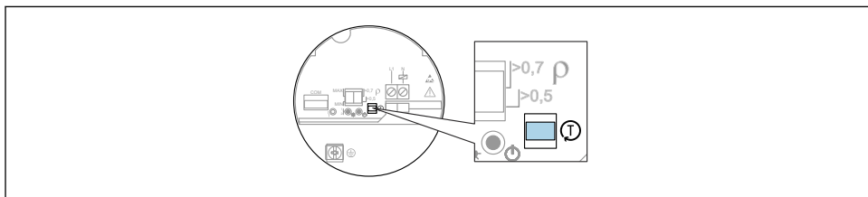
30 Nøkkelplassering for funksjonsprøving for elektronikkinnsetser FEL61/62/64/64DC/67/68
