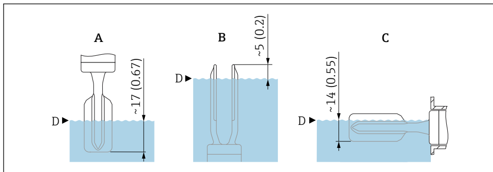
3 Typiske koblingspunkter, emaljebelagt stemmegaffel. Måleenhet mm (in)
