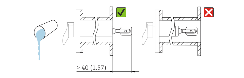
5 Installasjonseksempel for en svært viskøs væske. Måleenhet mm (in)
