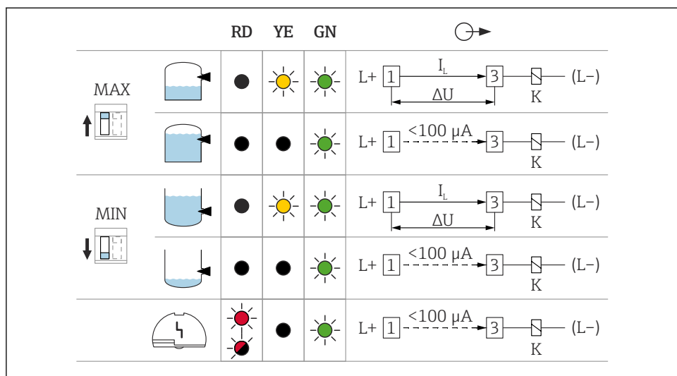
17 Koblingsutgangens og signaliseringens atferd, elektronikkinnsett FEL62
