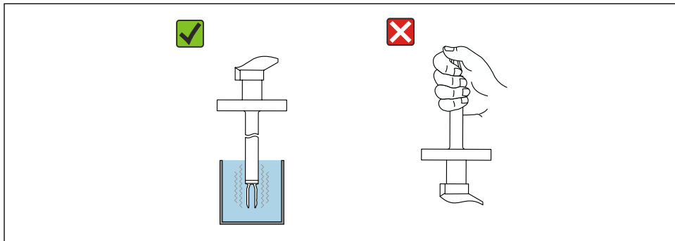
29 Funksjonstest av stemmegaffel
