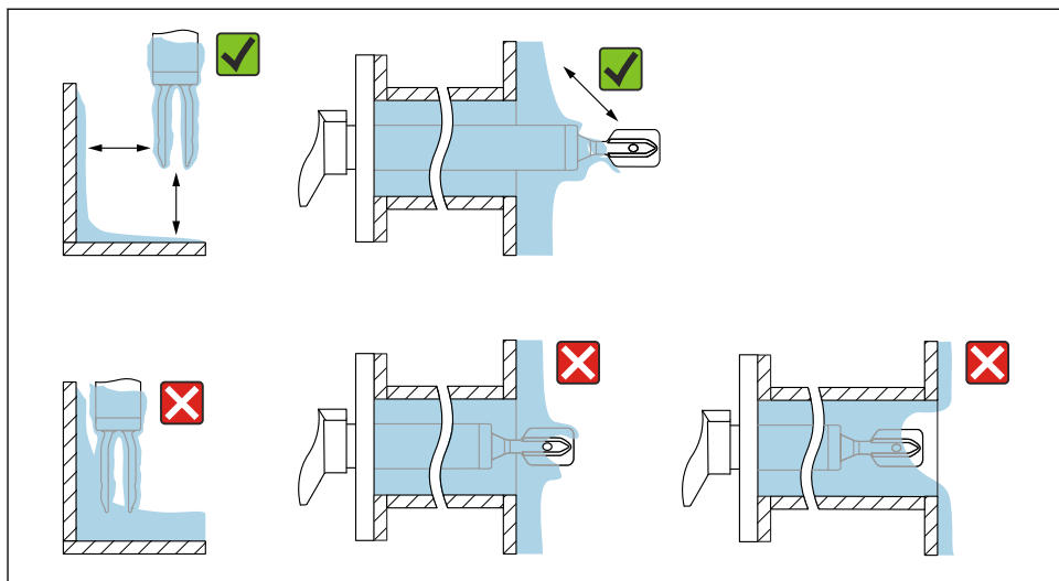
6 Installasjonseksempler for et svært viskøt prosessmedium
