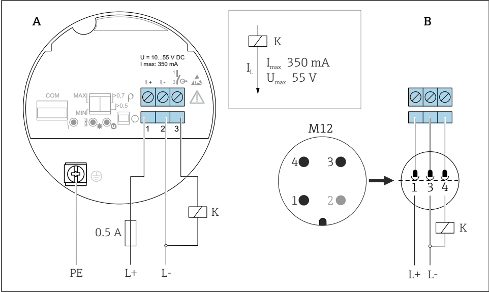
16 3-tråds DC-PNP, elektronikkinnsett FEL62
