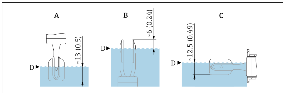
2 Typiske koblingspunkter, plastbelagt stemmegaffel (ECTFE, PFA). Måleenhet mm (in)
