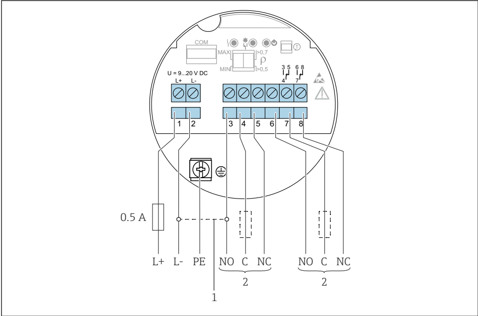
20 Likestrømstilkobling med reléutgang (elektronikkinnsats FEL64 DC)
