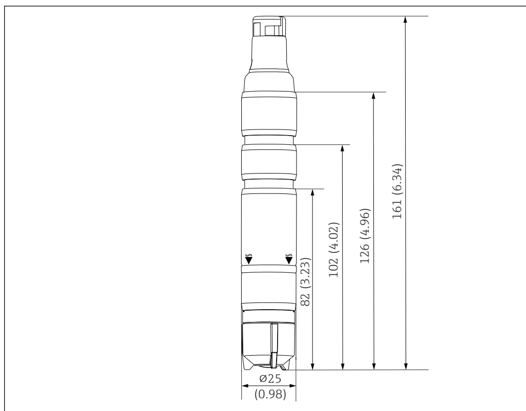
4 Mål i mm (tommer)
