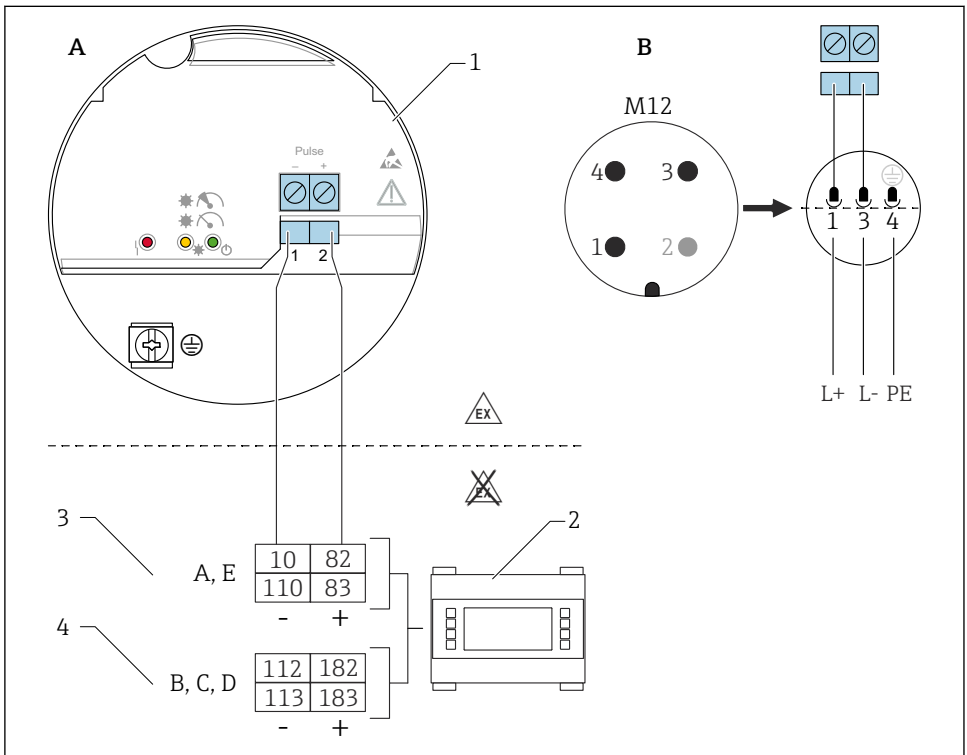
15 연결도: FEL60D 기판을 Density Computer FML621에 연결
