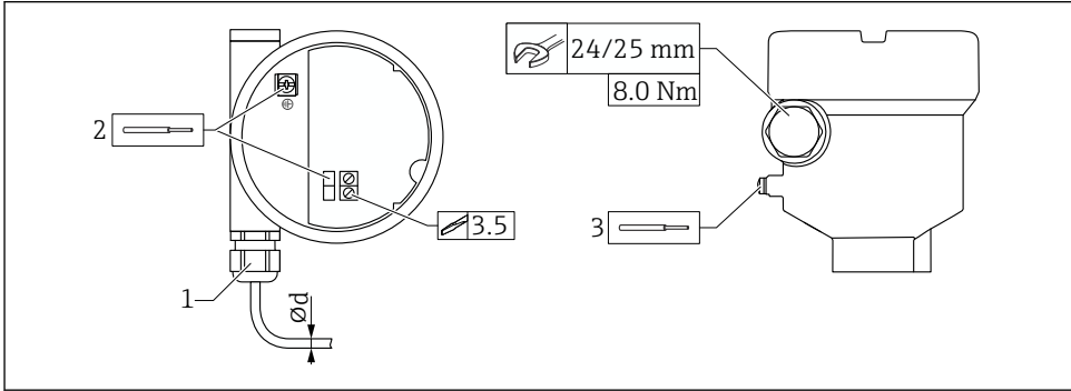
☞ 17 케이블 인입구 포함 커플링, 단자 포함 기판의 예
