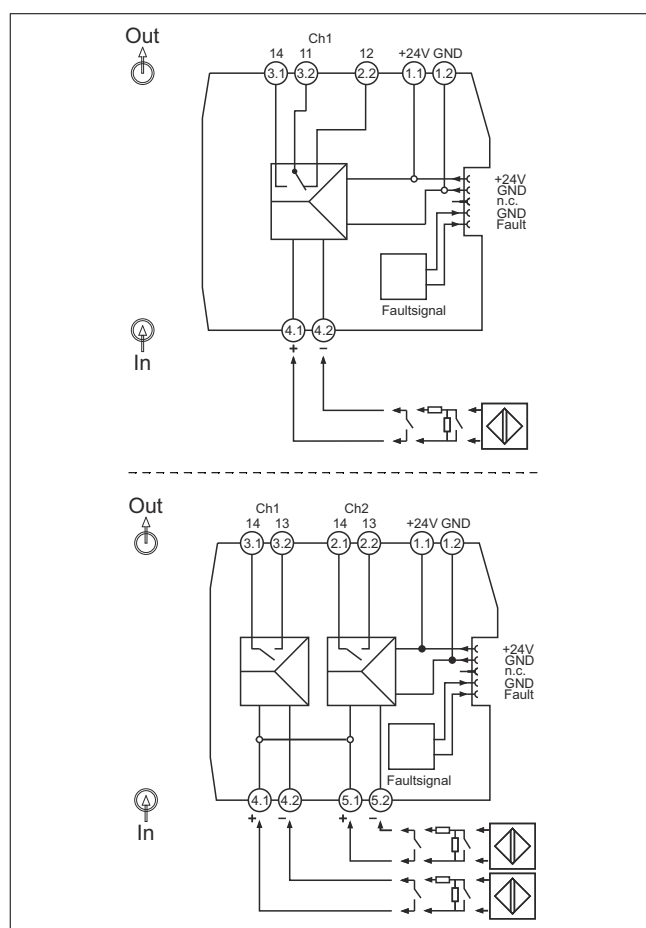
3 Připojení terminálu RLN22: 1kanálová verze (nahore), 2kanálová verze (dole)
