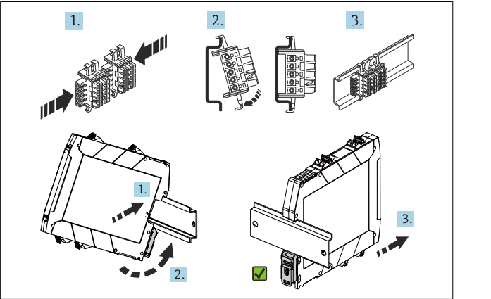
図 1 DIN レールバスコネクタ 12,5 mm (0,5 in) (上部) の取付けおよび DIN レール (下部) への取付け
