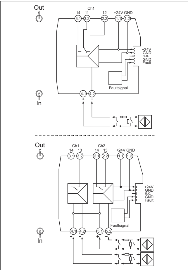
図 3 RLN22 の端子の割当て : 1 チャンネルバージョン (上)、2 チャンネルバージョン (下)
