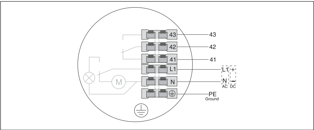
2 Assegnazione dei morsetti per l'interruttore di livello
