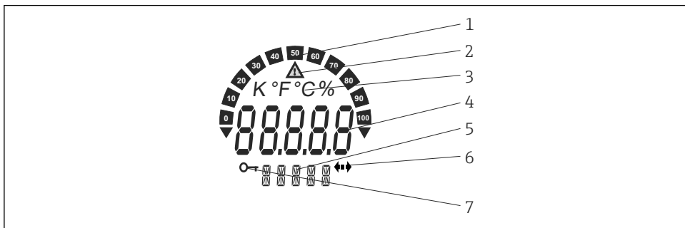
8 Wyświetlacz ciekłokrystaliczny przetwornika obiektowego (podświetlany, obracany co 90°)
