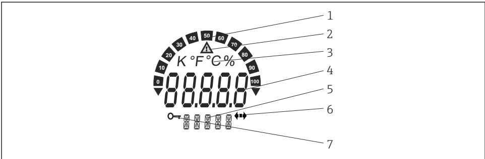
☐ 8 필드 트랜스미터의 LC 디스플레이(조명, 90° 단계로 연결 가능)
