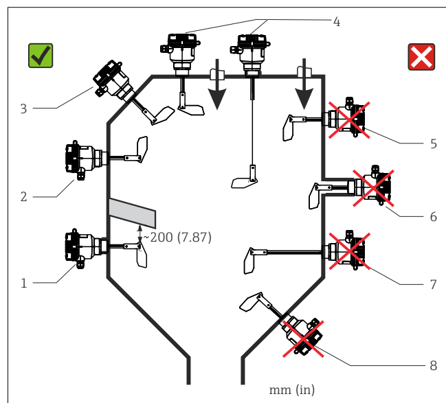
1 Correcte en verkeerde inbouwpositie van het instrument
