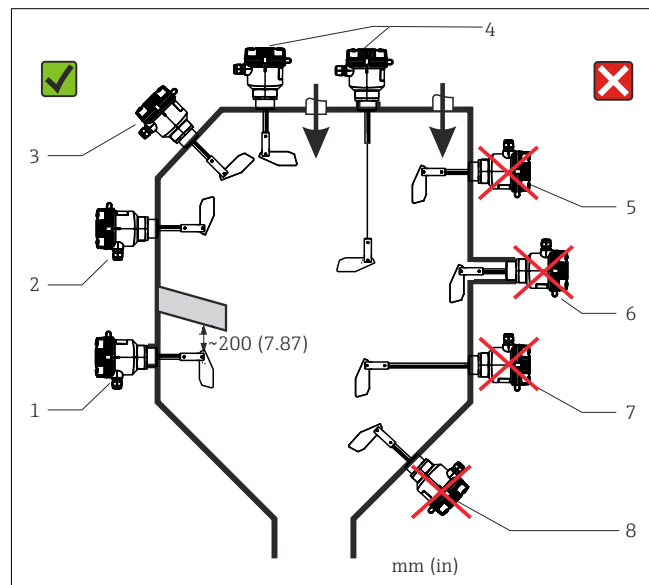
1 Orientamento corretto e scorretto del dispositivo
