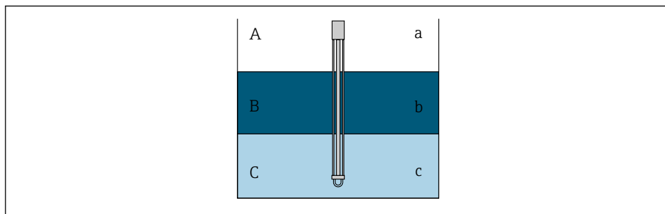
13 Waterniveaumeting in drie lagen
