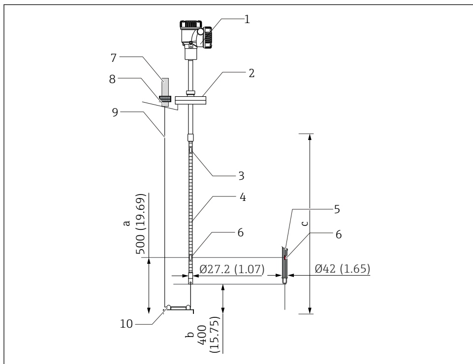
22 Topankermethode. Maateenheid mm (in)
