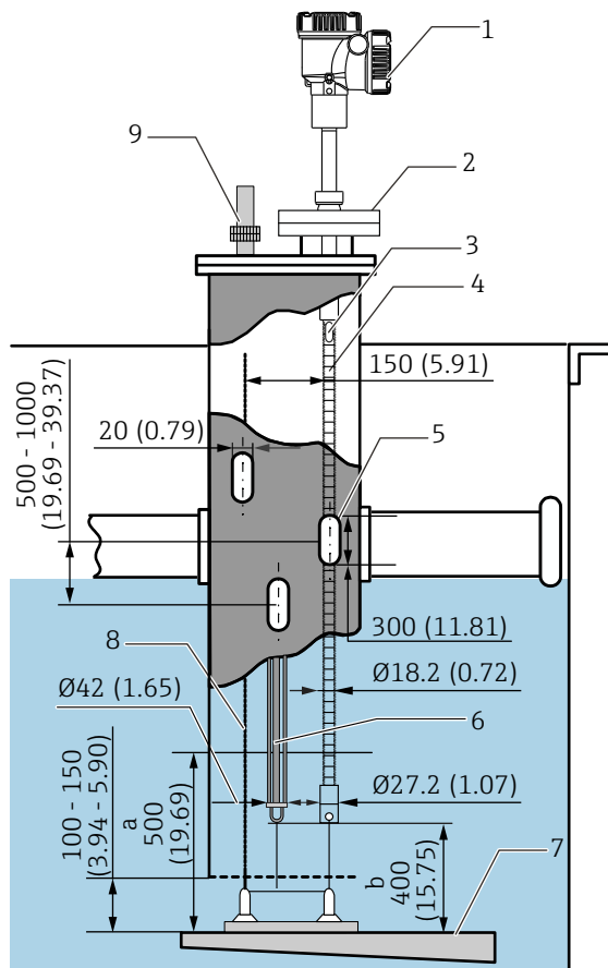
28 Topankermethode. Maateenheid mm (in)
