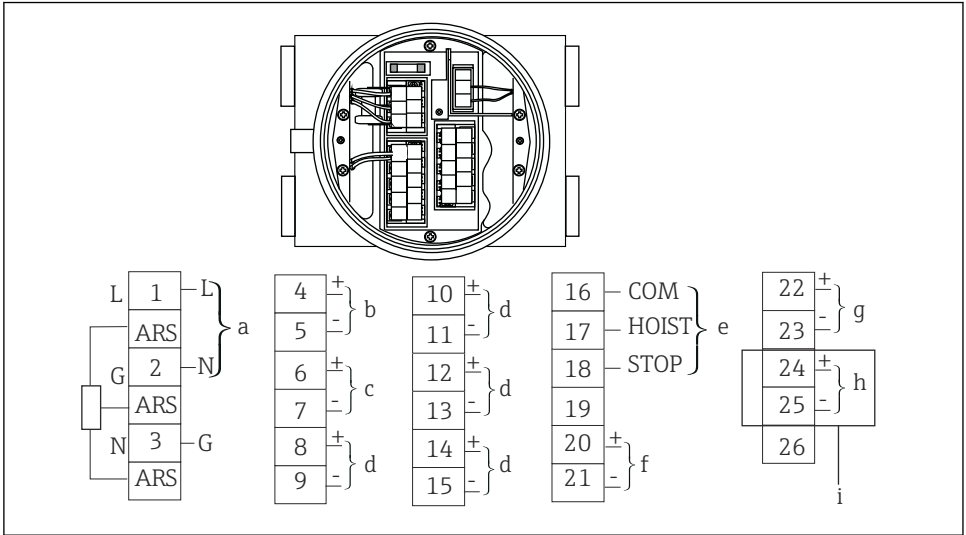
36 NMS5 klemmen
