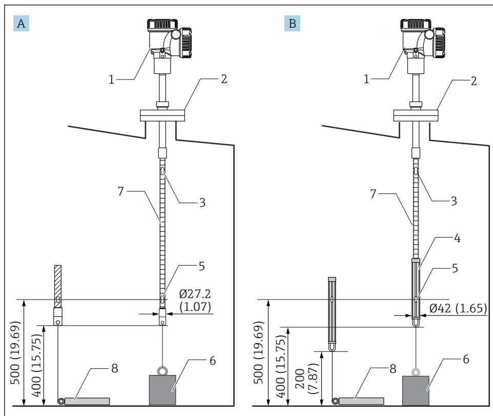
26 Ankergewichtmethode. Maateenheid mm (in)
