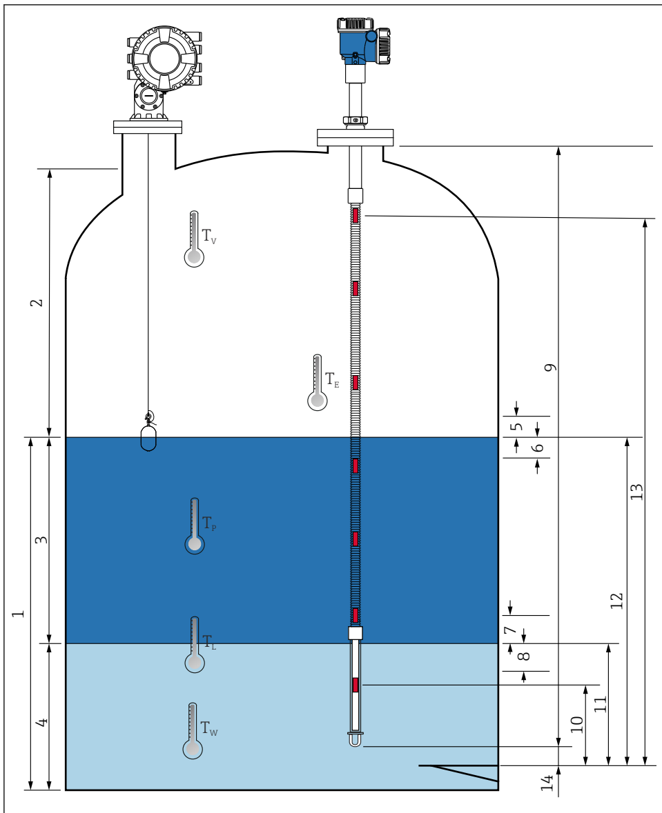
38 Terminologie gerelateerd aan NMT81 installatie
