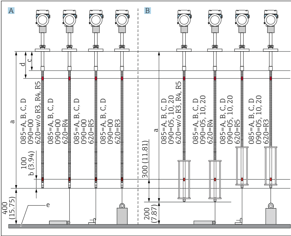
10 Positie van NMT81 elementnr. 1 afhankelijk van de installatiemethode. Maateenheid mm (in)
