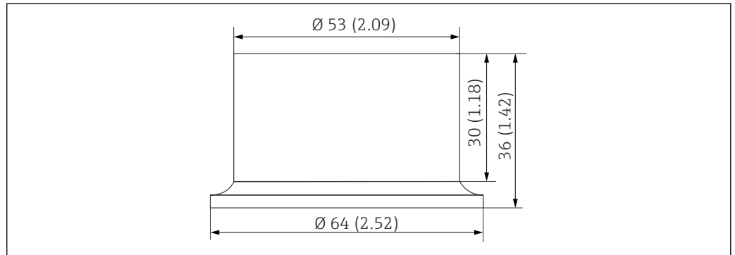
17 Приварной переходник. Размеры в мм (дюймах)
