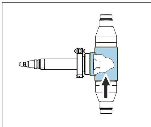
9 Монтаж с проточной арматурой CUA252
