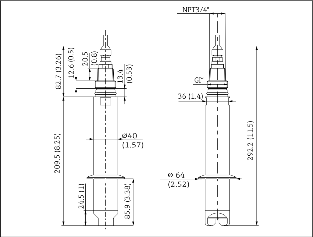
15 Размеры с зажимом. Размеры в мм (дюймах)
