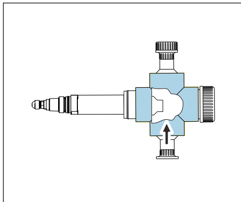
11 Монтаж с проточной арматурой CUA251
