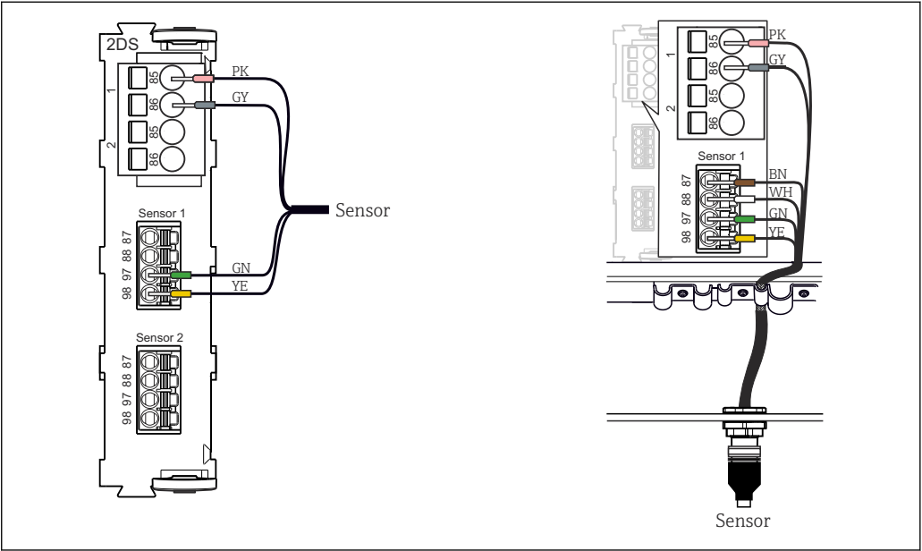
13 Подключение датчика к входу датчика (слева) или через разъем M12 (справа)
