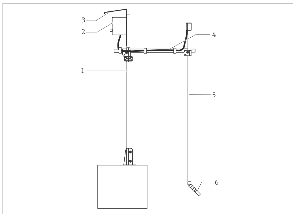
8 Измерительная система с погружной арматурой (пример)
