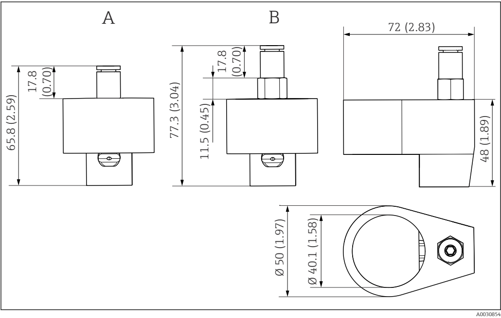
21 Система очистки сжатым воздухом. Единица измерения: мм (дюйм)
