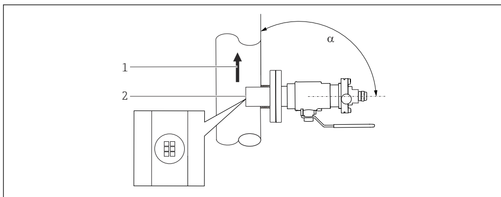
16 Монтаж с выдвижной арматурой
