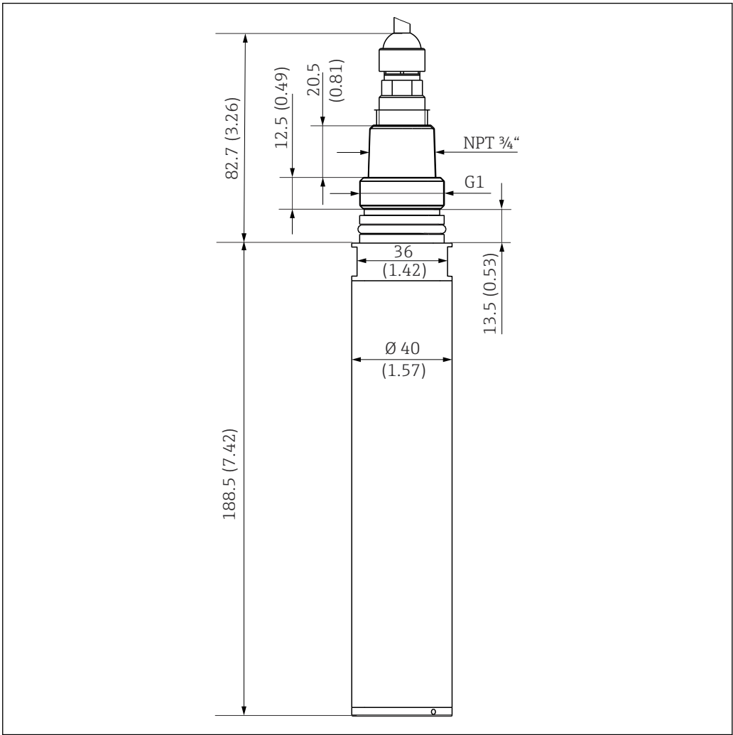
20 Размеры. Единица измерения: мм (дюйм)
