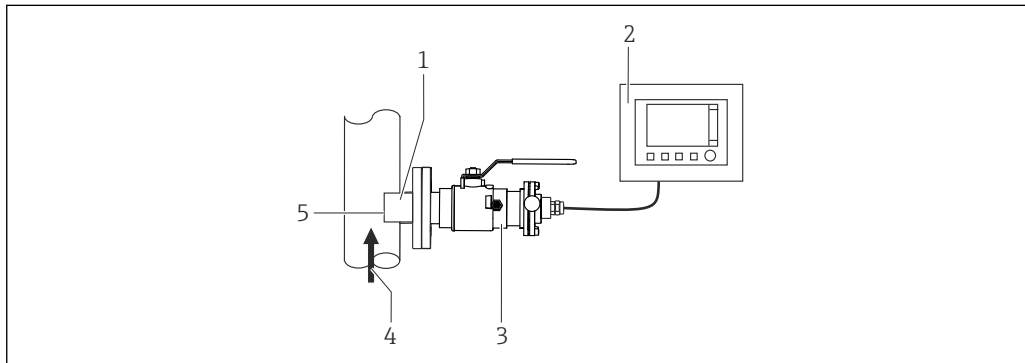
10 Измерительная система с выдвижной арматурой (пример)
