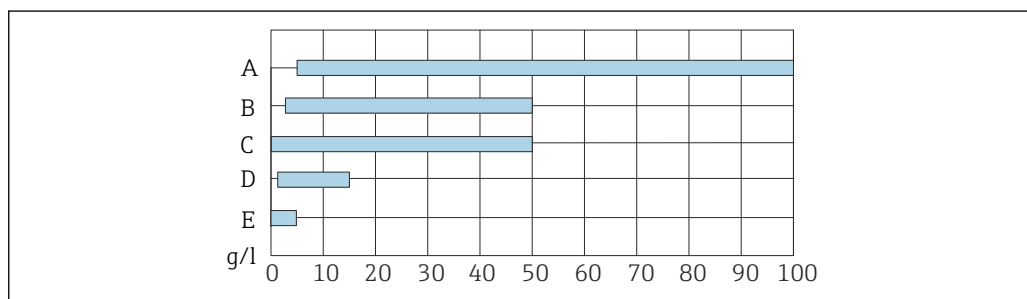
15 Среда: «твердые частицы»
