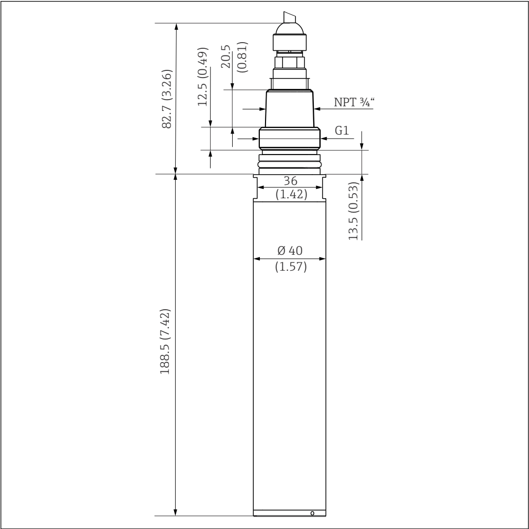
20 外形尺寸示意图；单位：mm (in)
