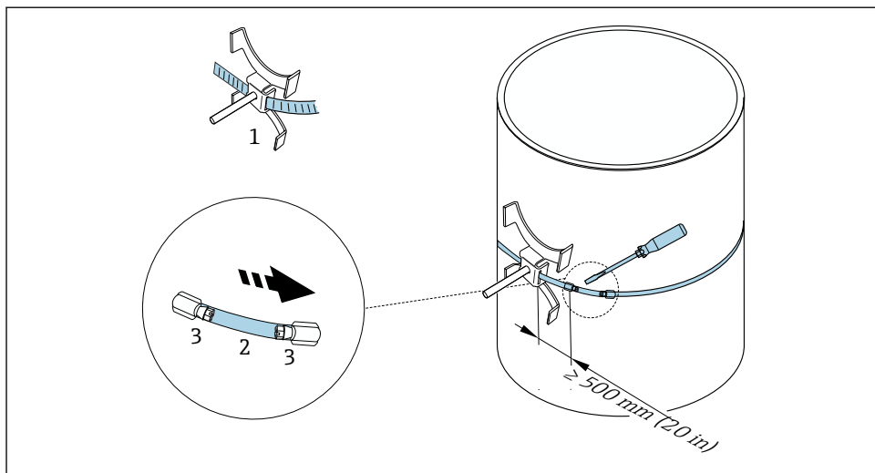
11 Houder met bevestigingsbanden (grote nominale diameters)
