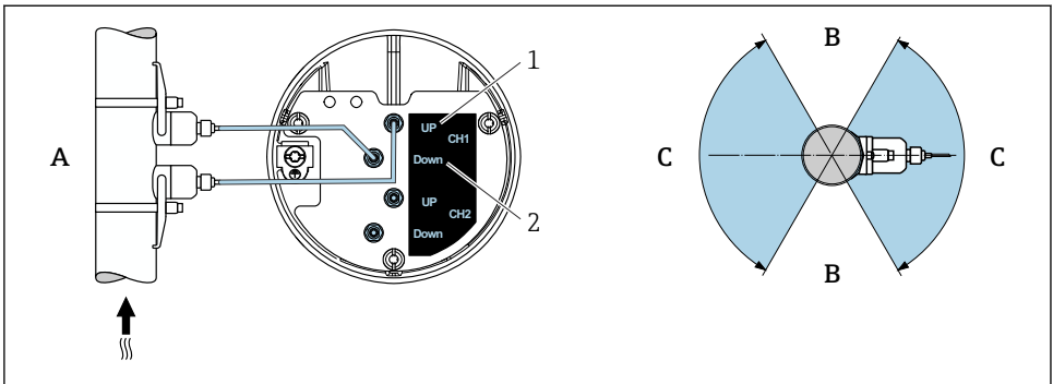
2 Inbouwpositie aanzichten
