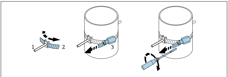
▣ 10 Houder met bevestigingsbanden (gemiddelde nominale diameters), zonder scharnierende schroef
