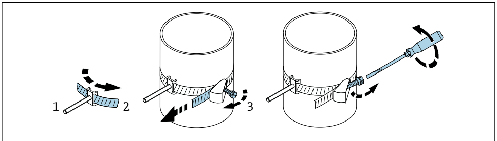
▣ 9 Houder met bevestigingsbanden (gemiddelde nominale diameters), met scharnierende schroef
