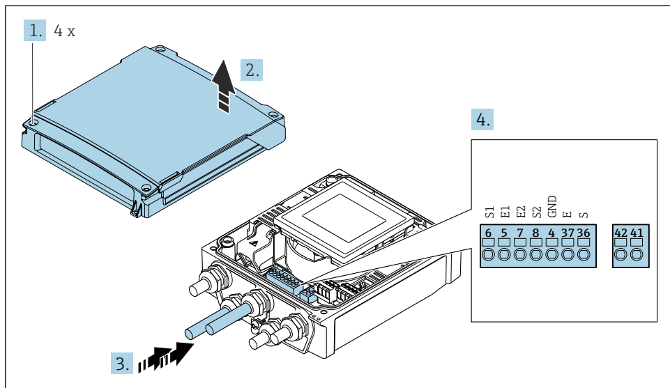
4 Transmitter: hovedelektronikmodul med klemmer
