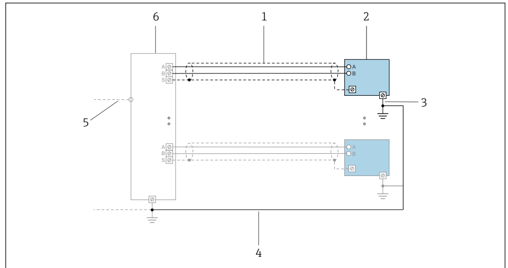
Fig. 16 Ejemplo de conexión para PROFINET con Ethernet APL
