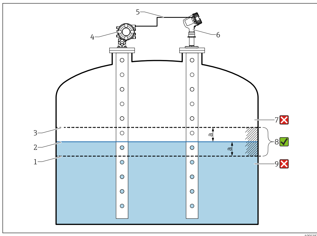
■ 22 Esempio di applicazione con Proservo NMS8x
