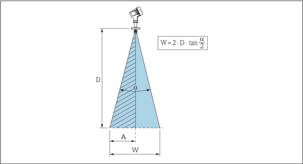
12 Rapporto tra angolo di emissione \alpha , distanza D e diametro del lobo di emissione W . La distanza A è la distanza minima dalla parete del serbatoio (o altre installazioni). La distanza A equivale alla metà del diametro del lobo di emissione W
