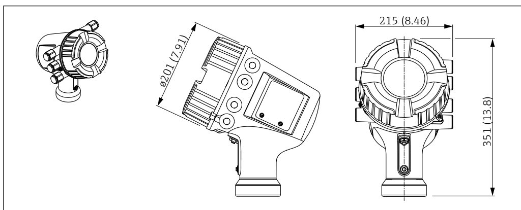
14 Dimensioni della custodia dell'elettronica; unità di misura: mm (in); in questo schema non sono considerati gli adattatori per gli ingressi cavo.
