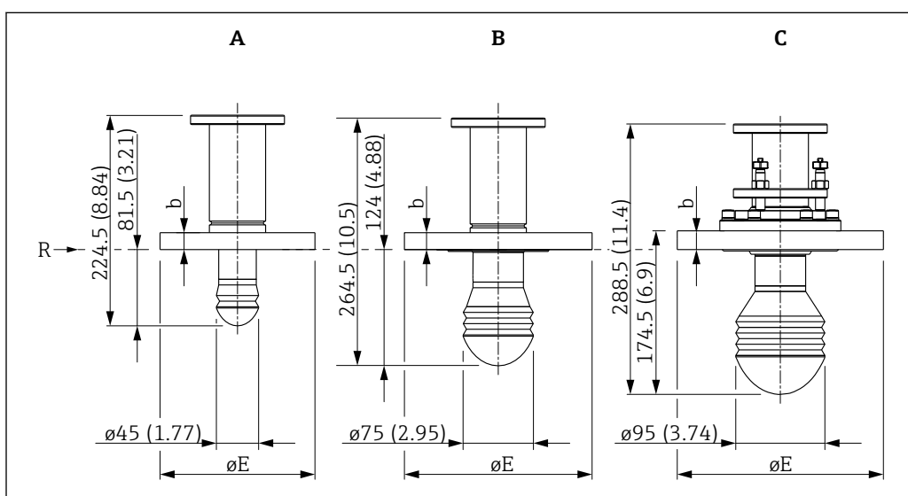
15 Dimensioni antenna; unità di misura: mm (in)
