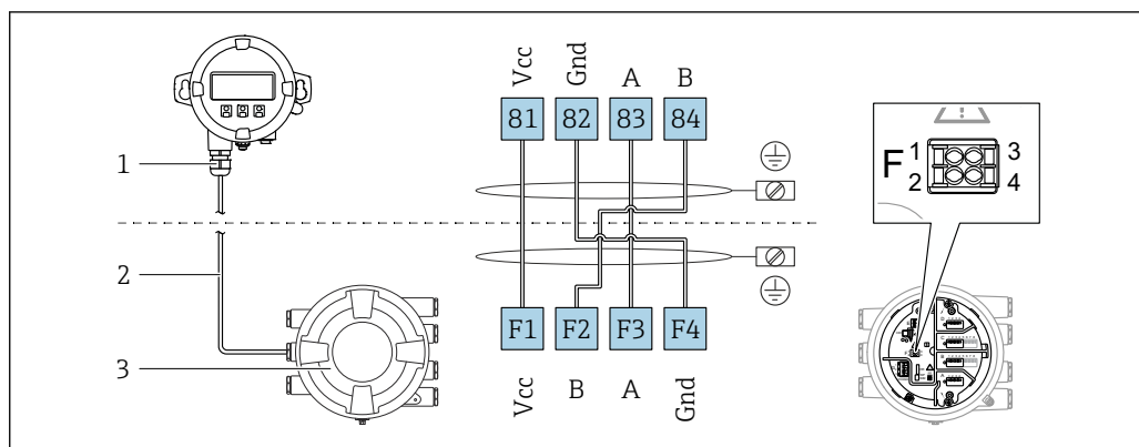
11 Connessione del modulo operativo e di visualizzazione separato DKX001 al dispositivo per la misura nei serbatoi (NMR8x, NMS8x o NRF8x)
