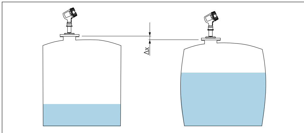
21 Movimenti \Delta x del livello di riferimento che si generano per la deformazione delle pareti del serbatoio causata dalla pressione idrostatica
