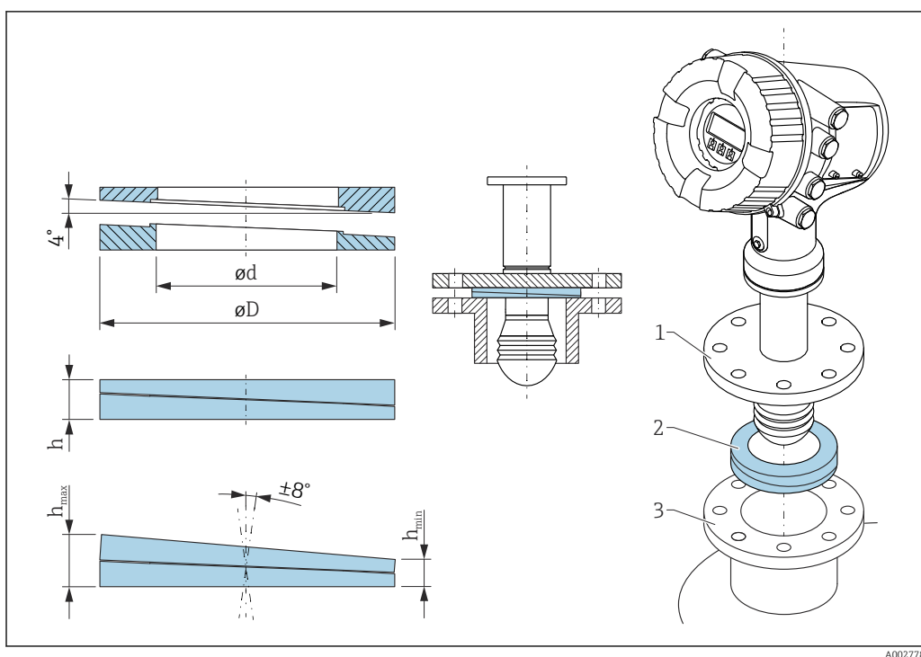
26 Tenuta regolabile usata per orientare il dispositivo di \pm 8^\circ
