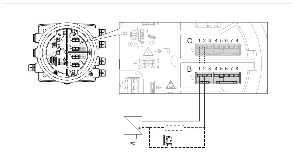
7 Ingresso o uscita passivi: usare i morsetti 1 e 2
