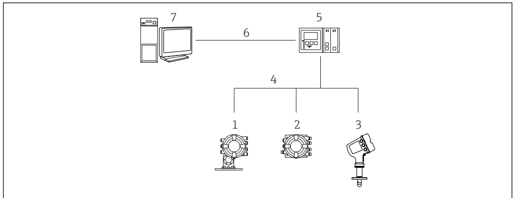
19 Comando a distanza dei dispositivi di misura nei serbatoi
