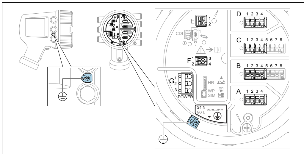
9 Vano morsetti (esempio tipico) e morsetti di terra
