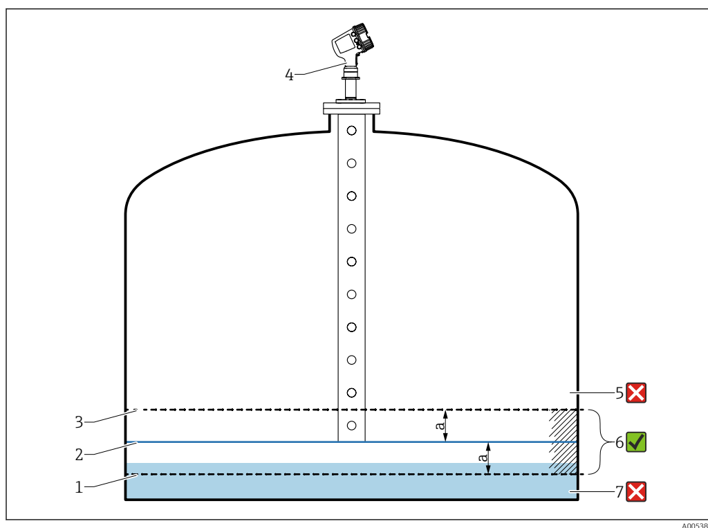
23 Esempio di applicazione con punto di riferimento fisso all'estremità del tubo di calma
