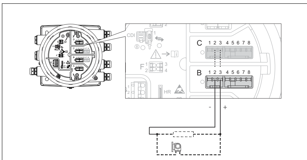
8 Ingresso o uscita attivi: usare i morsetti 2 e 3
