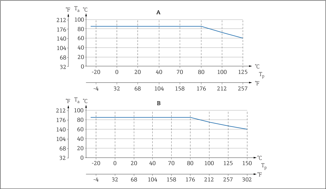
9 Les valeurs sont valables pour un montage vertical sans isolation. A Toutes les versions sauf B B "Version haute température" Tp Température de process Ta Température ambiante
