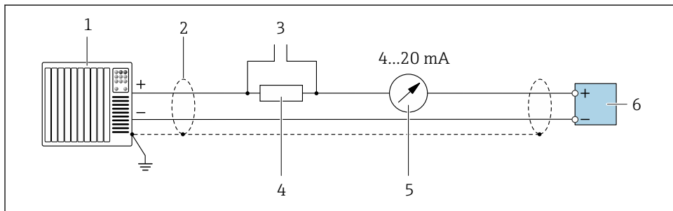
5 Exemplu de conexiune pentru ieșire curent între 4 și 20 mA HART (activă)
