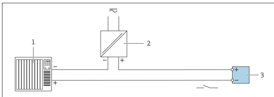
12 Exemplu de conexiune pentru ieșire releu (pasivă)
