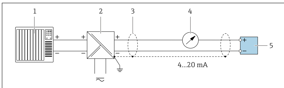
6 Exemplu de conexiune pentru ieșire curent între 4 și 20 mA HART (pasivă)
