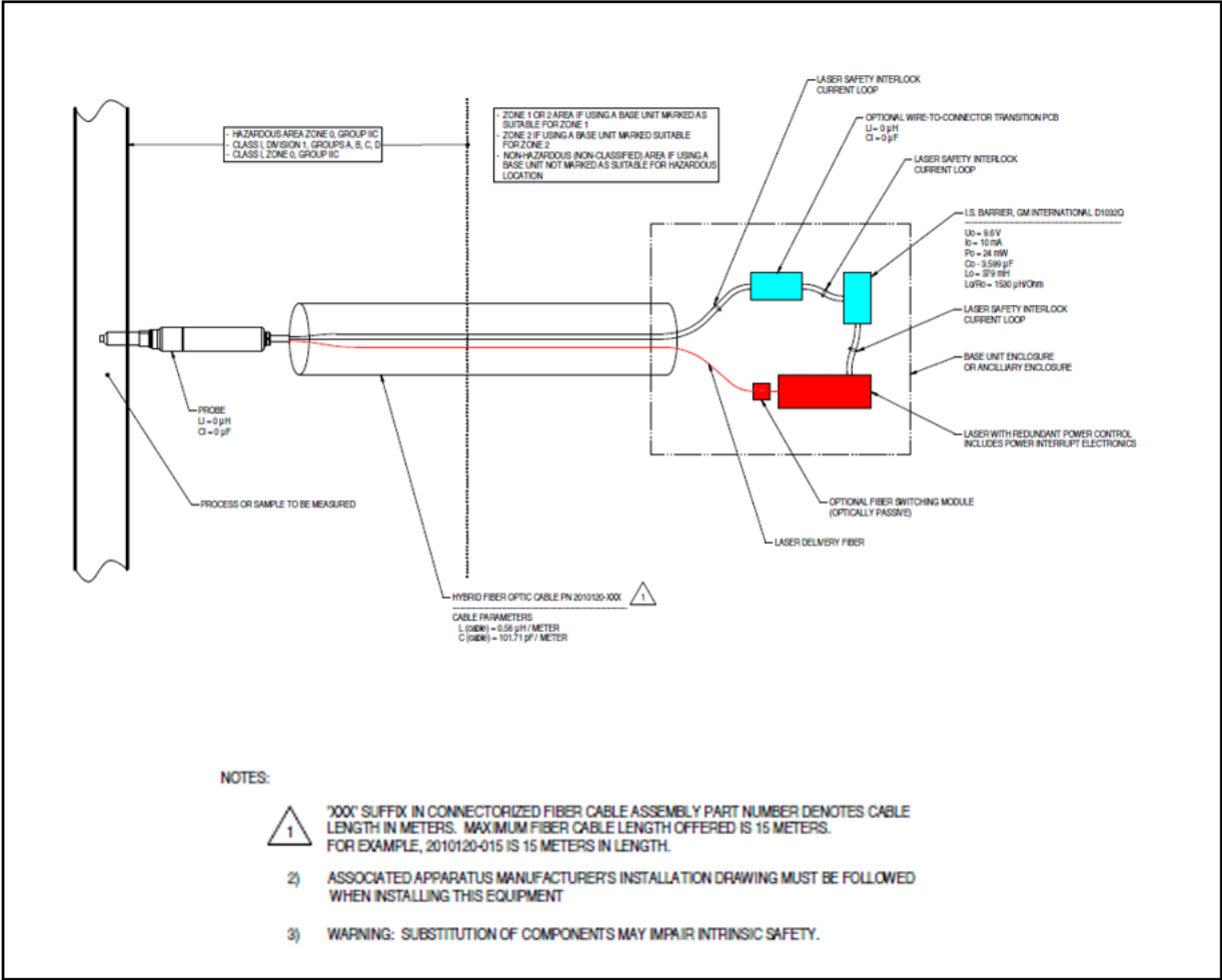
图 9. Rxn-20 防爆危险区安装图示 (3000272 X2)
