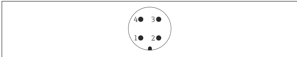
19 M12 priključak, dodjela pinova
