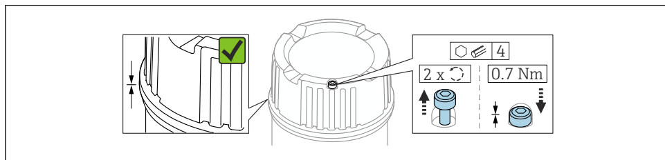
15 Poklopac sa vijkom za pričvršćivanje
