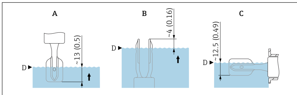
2 Značilne točke preklopa. Merska enota mm (in)
