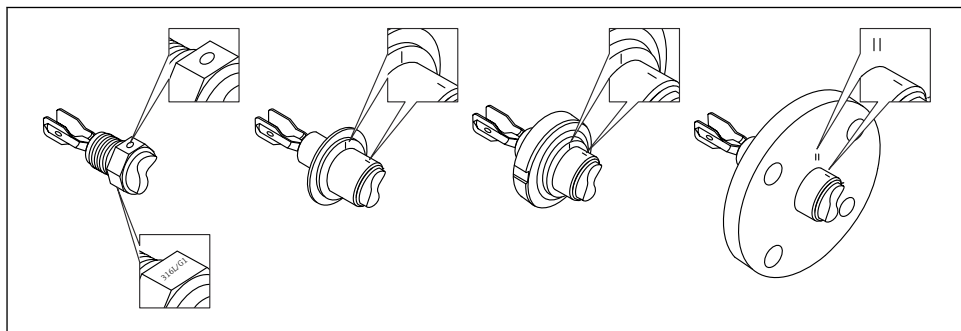
9 Posición del diapasón en caso de instalación horizontal en el depósito usando el marcado
