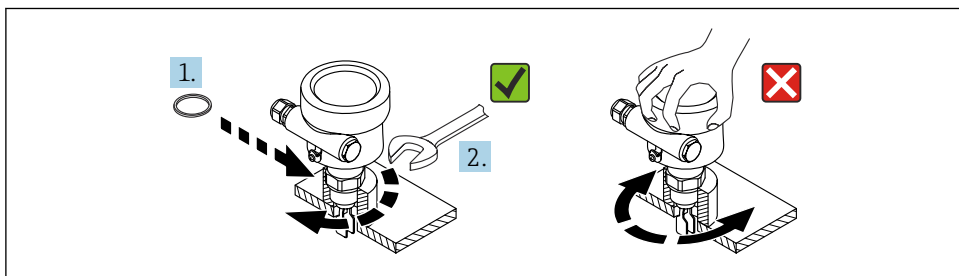
11 Enroscado del equipo
