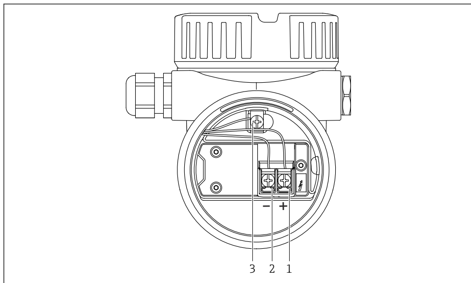
17 Terminales de conexión y borne de tierra en el compartimento de conexiones
