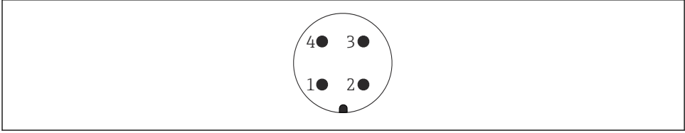
18 Conector M12, asignación de pines
