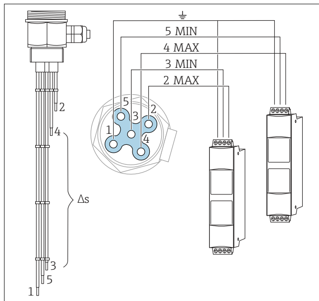
■ 3 接続例：5 本のロッドプローブを 2 つの評価ユニットに接続する場合
