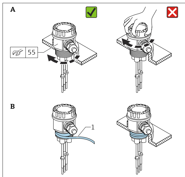
■ 2 機器の締め付け
