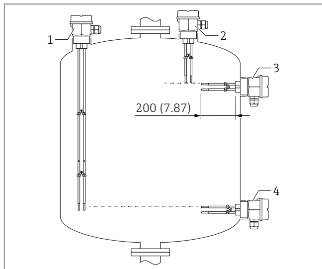
■ 1 タンク内のロッドプローブの位置
