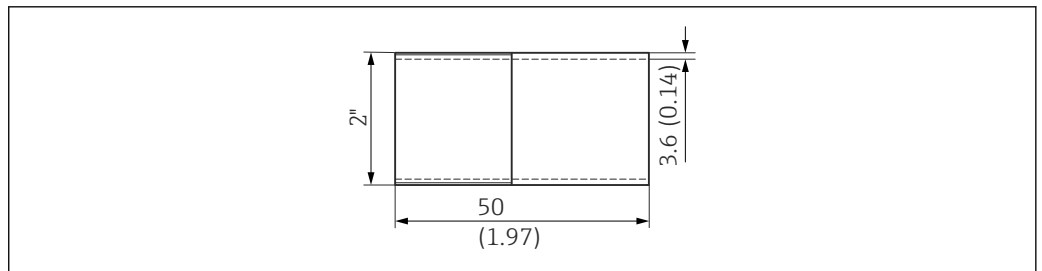
13 Króciec do spawania, wymiary w mm (calach)
