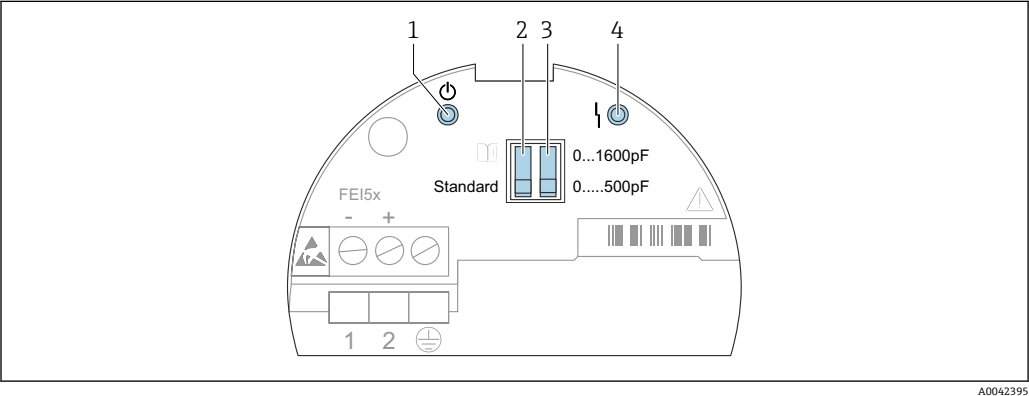
図 29 FEI53 と FEI57S のヒューマンインタフェース
