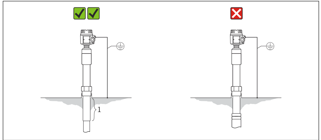
図 10 導電性のサイロ壁
