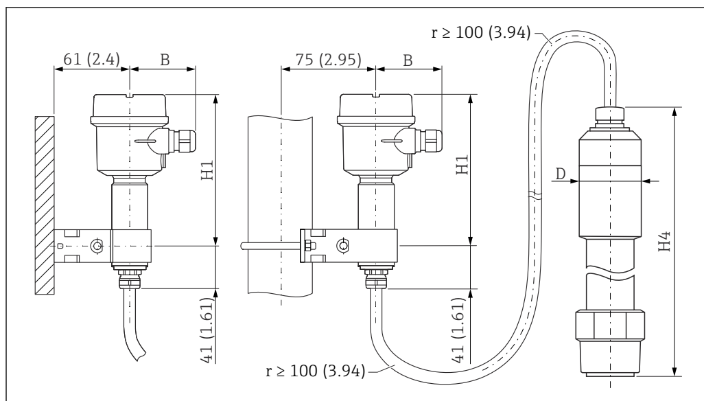
図 19 ハウジング側：壁面取付け、パイプ取付け、およびセンサ側。測定単位 mm (in)
