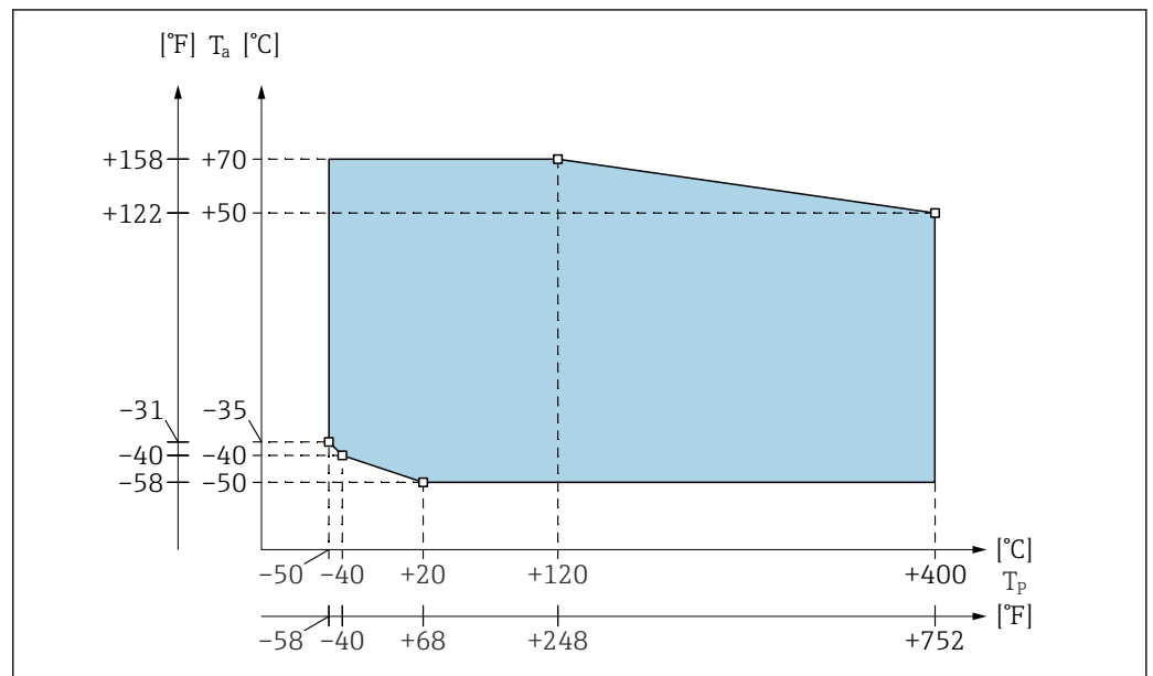
図 68 プロセス温度範囲図：ソード/ローププローブ
