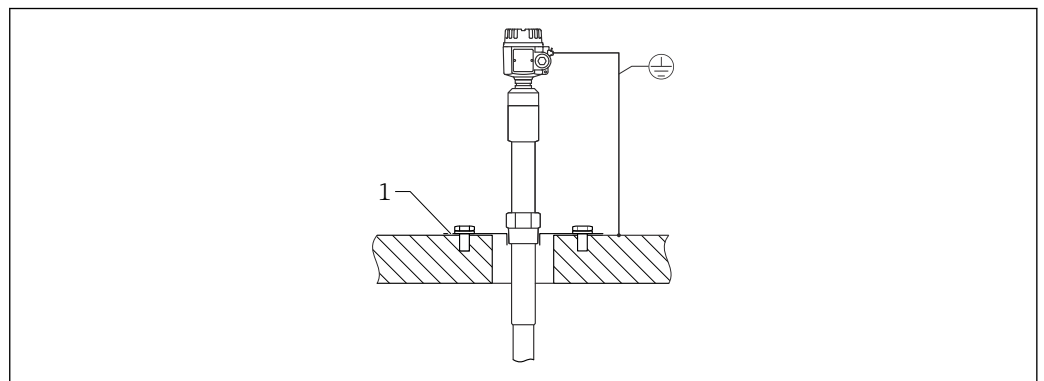
図 11 コンクリート製のサイロ壁
