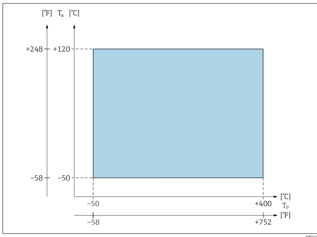
図 69 プロセス温度図：分離型ハウジング
