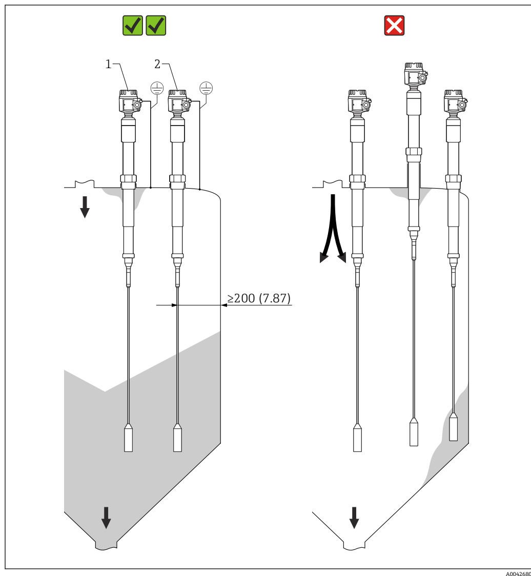
図 9 ローププローブの取付け例
