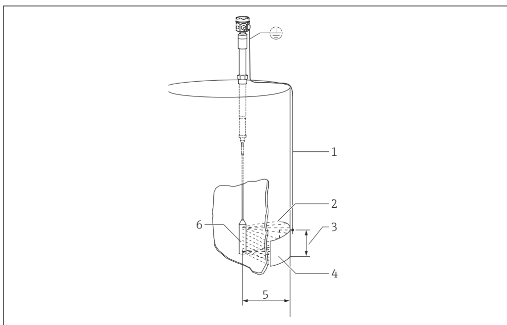
図 13 樹脂タンクへのプローブの取付け
