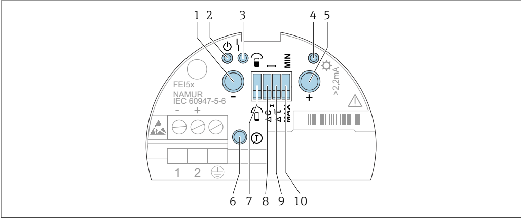
34 FEI58 のヒューマンインタフェース
