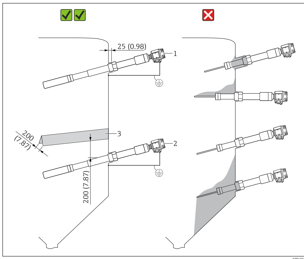
図 2 側面への取付例。測定単位 mm (in)
