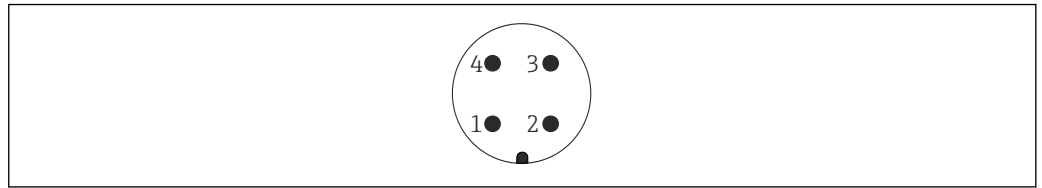
図 24 M12 コネクタ : 2 線式エレクトロニックインサート FEI55、FEI57、FEI58、FEI57C
