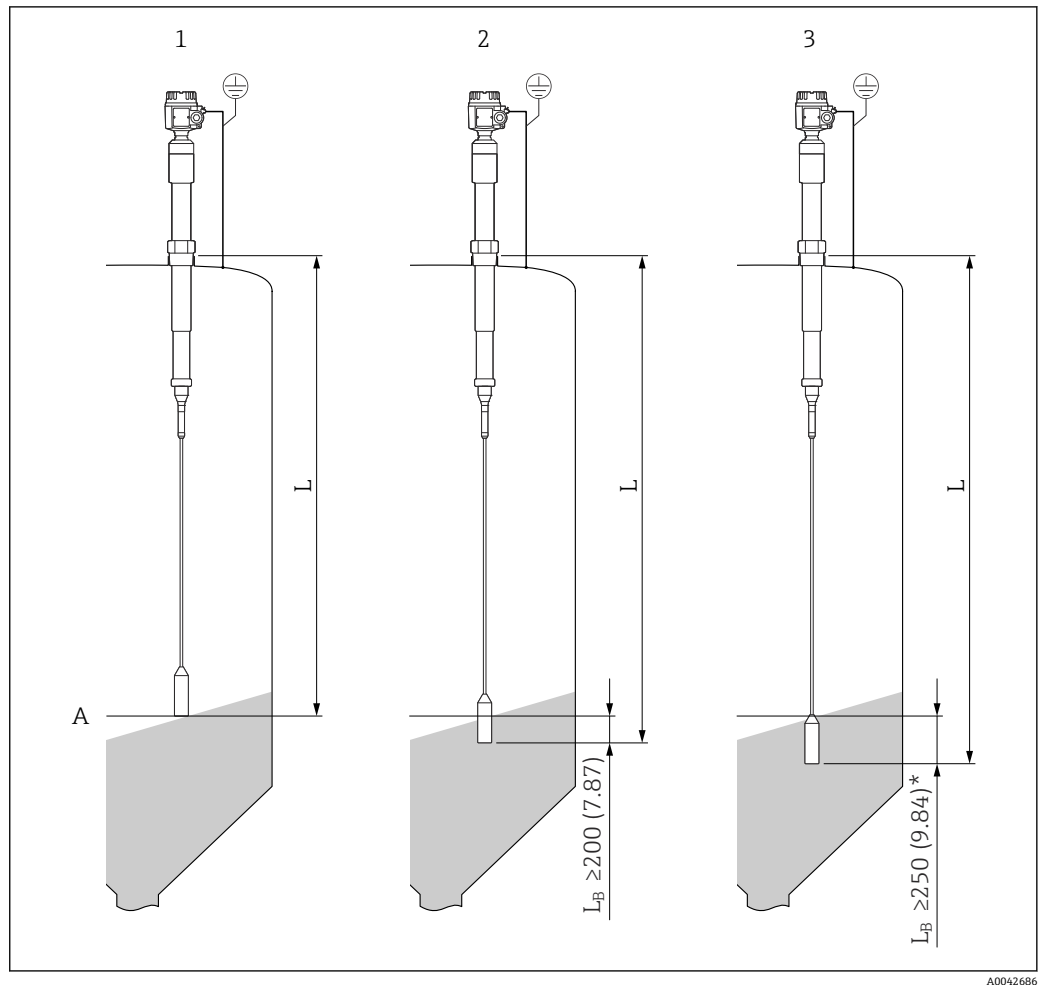
図 14 ロープ長と測定物の相関関係。測定単位 mm (in)
