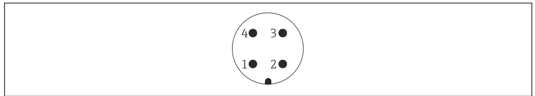
図 25 M12 コネクタ : 3 線式エレクトロニックインサート FEI52、FEI53
