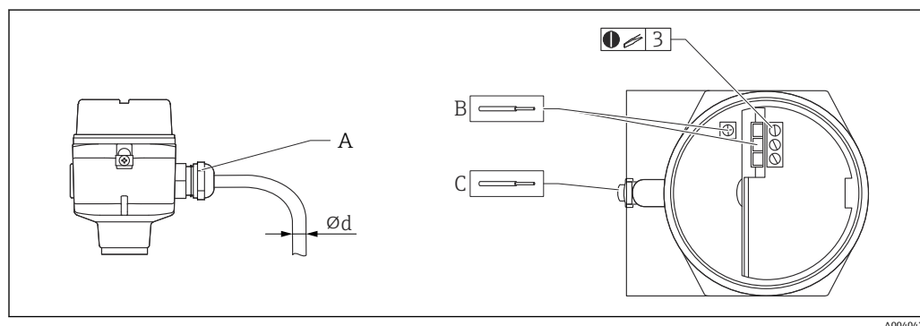
図 23 プローブおよびエレクトロニックインサート接続部
