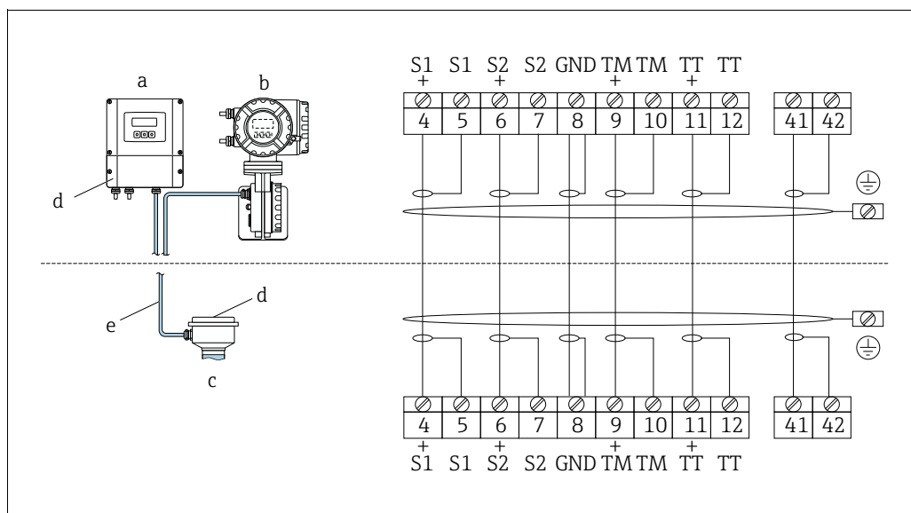
Fig. 17: Connexion câble de raccordement version séparée
