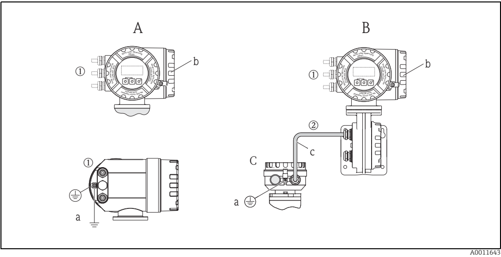
Abb. 3: Aufbau des Messsystems Kompakt-/Getrenntausführung
