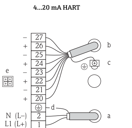
Fig. 18: Raccordements électriques
