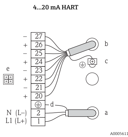
Abb. 6: Elektrische Anschlüsse
