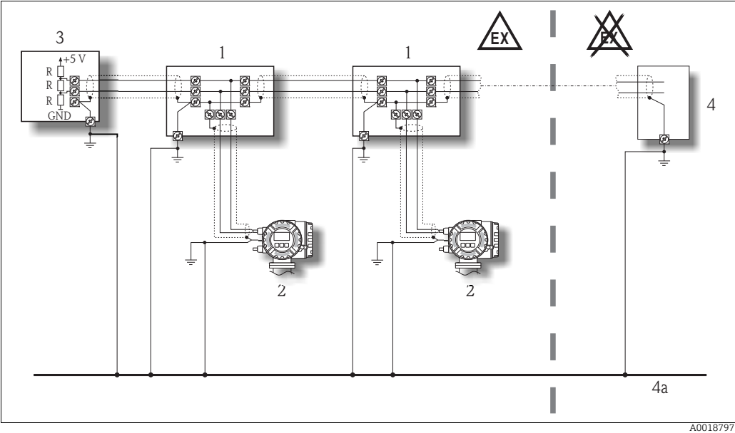
Abb. 2: Beispiel für den Anschluss von Potentialausgleichsleitungen
