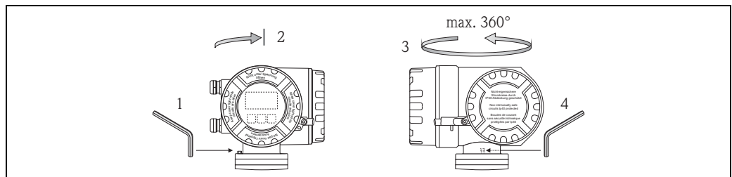
Abb. 1: Messumformergehäuse drehen
