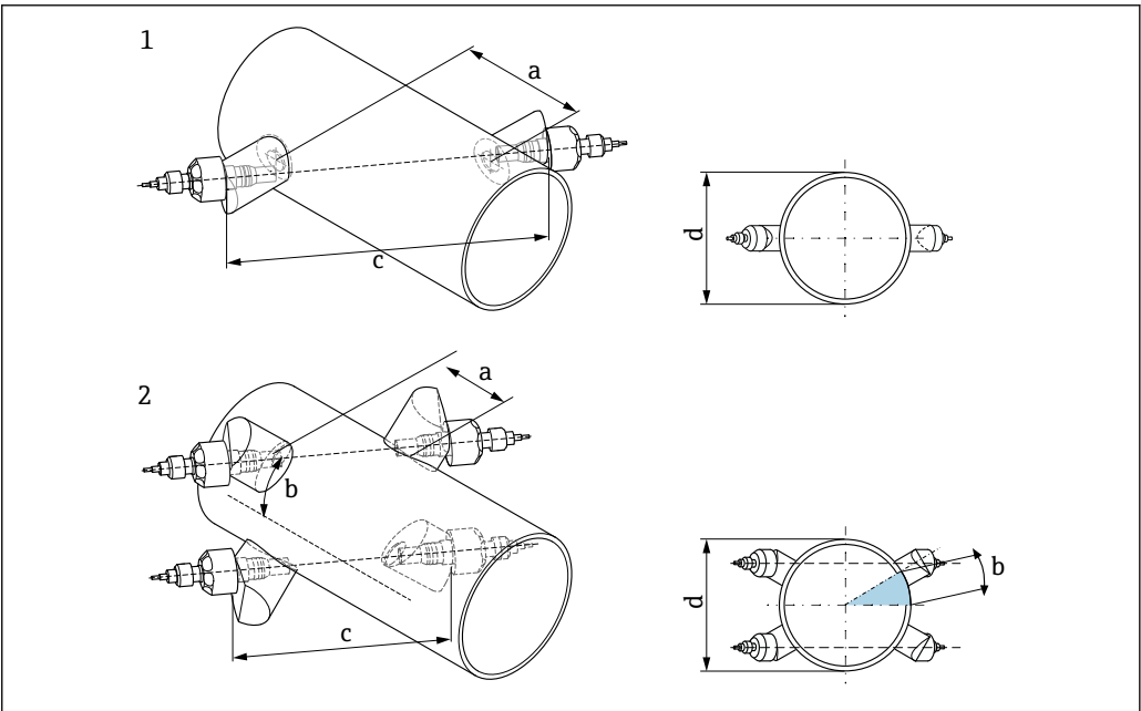
9 Descrizione della terminologia di installazione
