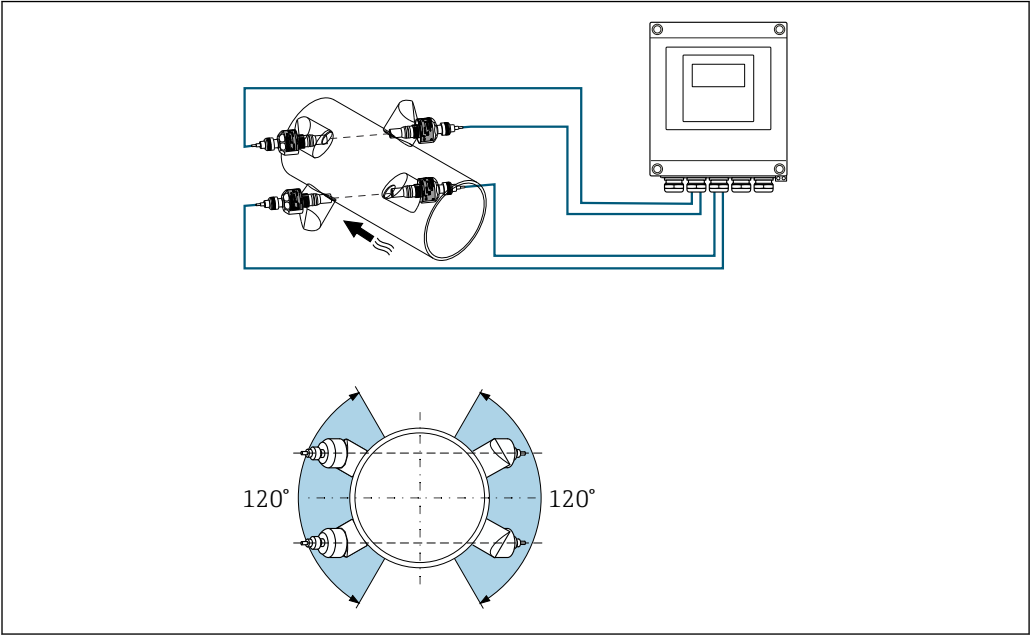
7 Misura a due vie: esempi di posizionamento orizzontale dei set di sensori al punto di misura
