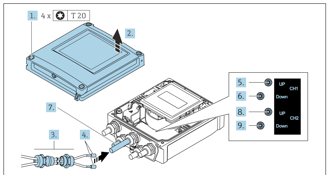
12 Trasmettitore: modulo dell'elettronica principale con morsetti
