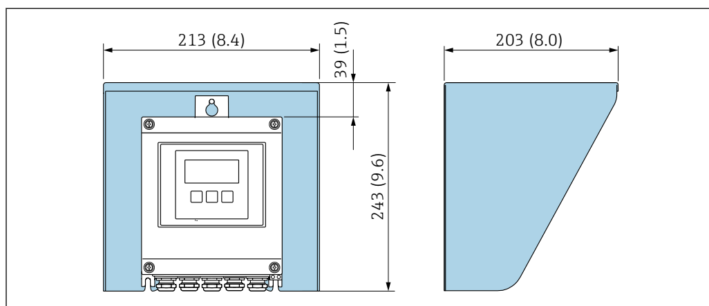
8 Tettuccio di protezione dalle intemperie, unità ingegneristiche mm (in)
