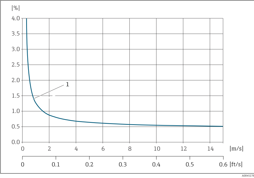
26 Esempio di errore di misura max (portata volumetrica) in % v.i. 1 Diametro del tubo ≥ 250 (10")
