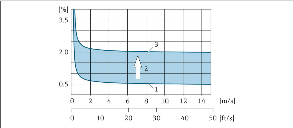
25 Esempio di errore di misura in un tubo con diametro nominale DN > 200 (8") 1 Errore di misura del misuratore: 0,5% v.i. ± 3 mm/s (0,12 in/s) 2 Errore di misura dovuto alle condizioni di installazione: tipicamente 1,5% v.i. 3 Errore di misura al punto di misura: 0,5% v.i. ± 3 mm/s (0,12 in/s) + 1,5% v.i. = 2% v.i. ± 3 mm/s (0,12 in/s)
