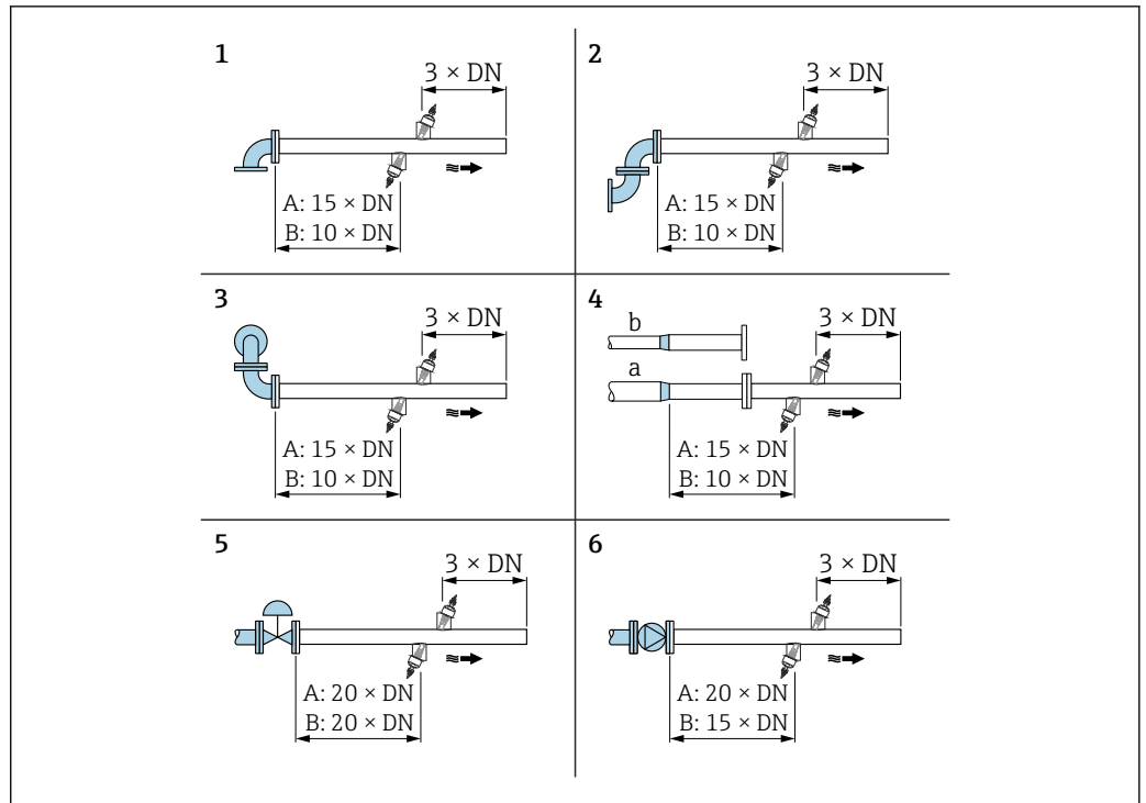
6 Tratti rettilinei minimi in entrata e in uscita per varie ostruzioni della portata (A: misura a una via, B: misura a due vie)
