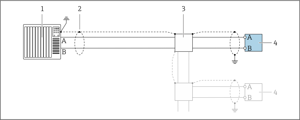
13 Esempio di connessione per Modbus RS485, area sicura e Zona 2/Div. 2 1 Sistema di controllo (ad es. PLC) 2 Schermatura del cavo di massa a un'estremità. La protezione del cavo deve essere messa a terra su entrambe le estremità per garantire la conformità alle prescrizioni EMC; osservare le specifiche del cavo 3 Scatola di distribuzione 4 Trasmettitore
