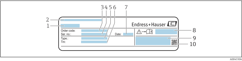
3 Esempio di targhetta del sensore, "anteriore"
