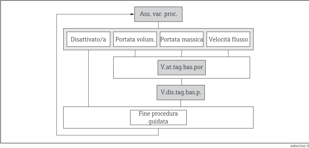
21 Procedura guidata "Taglio bassa portata" nel menu "Setup"
