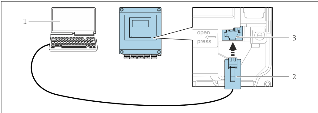
图 43 通过服务接口（CDI-RJ45）连接
