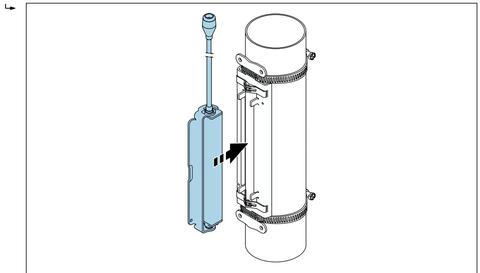
图 24 安装传感器外壳
