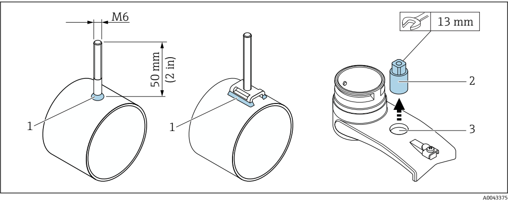
图 22 带焊接螺栓的传感器安装支座
