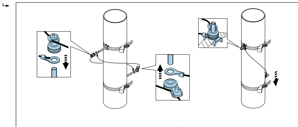
图 27 定位捆扎带（步骤 2...4）
