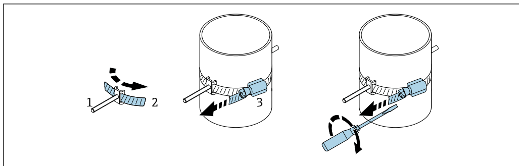
图 20 带捆扎带、不带铰接螺丝的传感器安装支座（中等公称口径）
