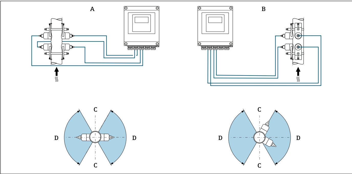
图 6 双声路测量：在测量点处水平布置传感器组的示意图
