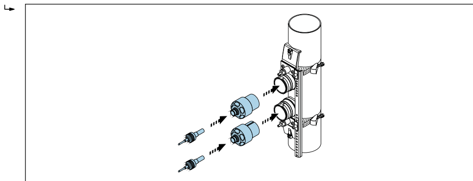
图 34 安装传感器并连接传感器电缆
