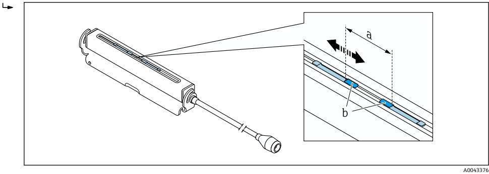
图 23 符合安装距离要求的传感器间距
