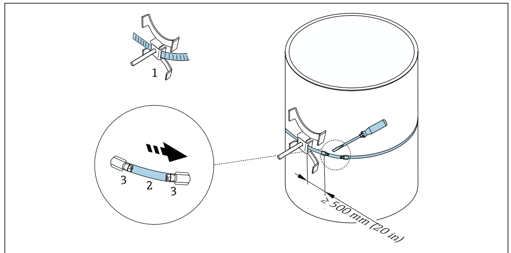
图 21 带捆扎带的传感器安装支座 (大公称口径)
