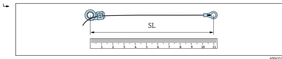
图 26 固定件与电缆接线头之间的距离等于测量线长度（SL）
