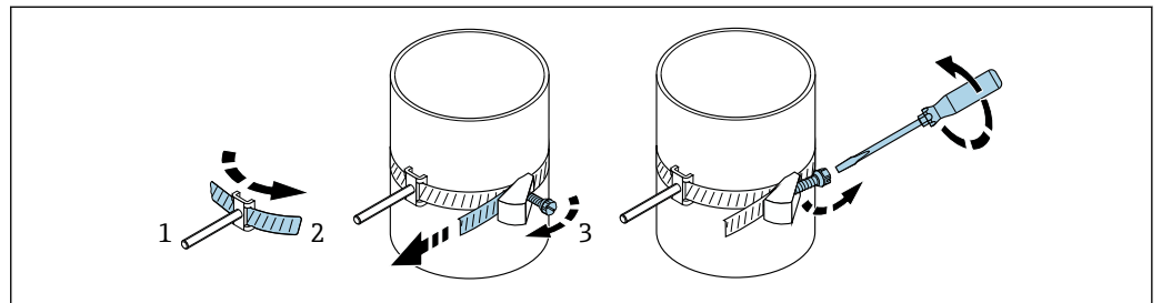
19 带捆扎带和铰接螺丝的传感器安装支座（中等公称口径）
