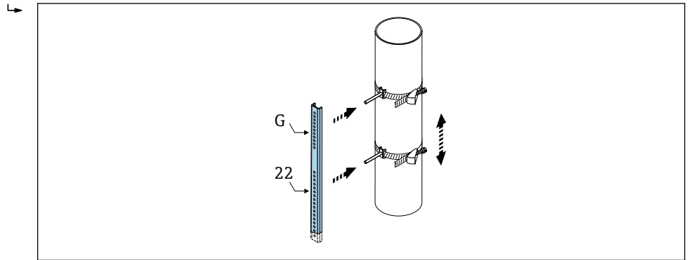
图 32 根据安装导轨确定距离 (例如 G22)。
