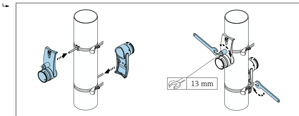
图 29 安装传感器安装支座
