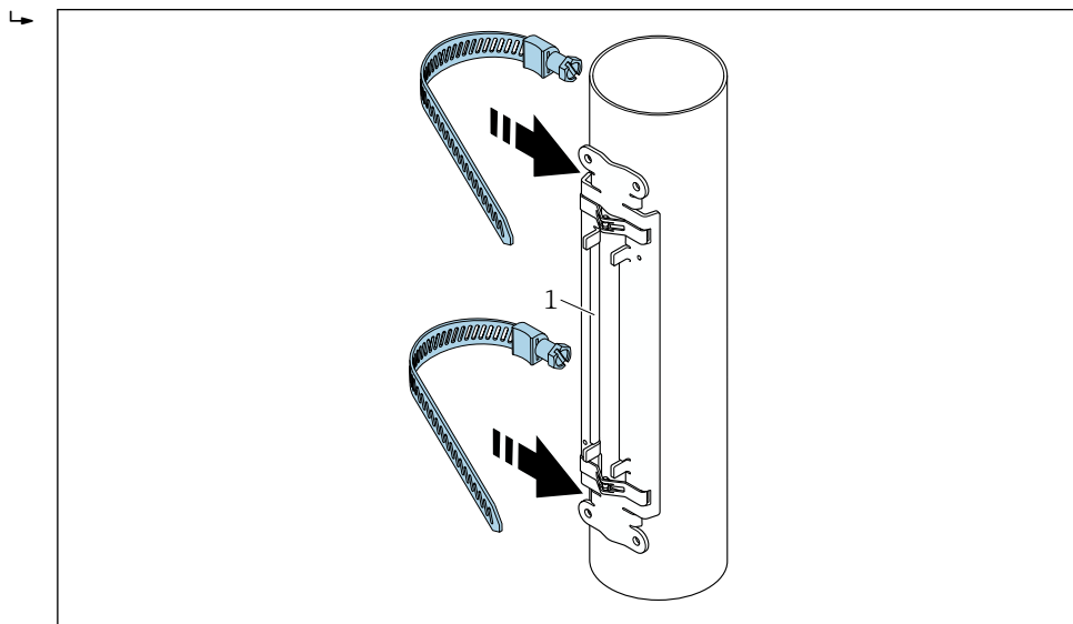
图 17 定位传感器安装支座并安装捆扎带。
