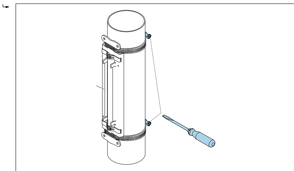
图 18 拧紧捆扎带的紧固螺丝。
