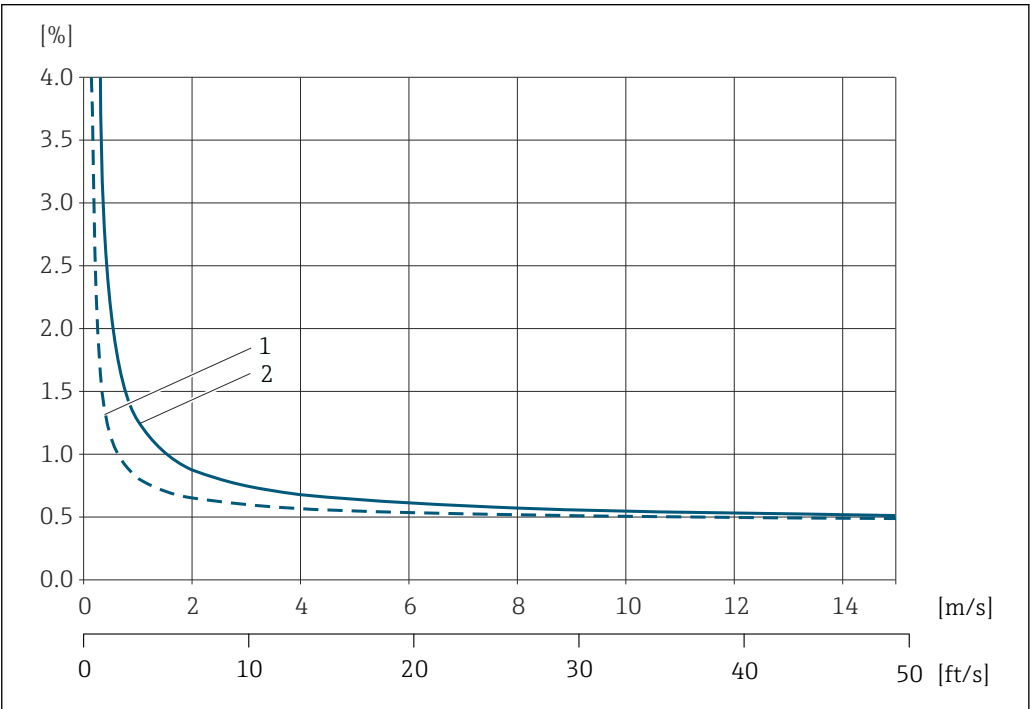
图 51 最大测量误差（体积流量）(% o.r.)的计算实例
