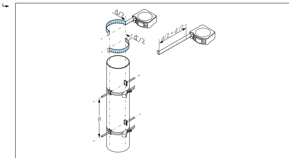
图 28 使用卷尺定位捆扎带和安装螺栓 (步骤 2...4)
