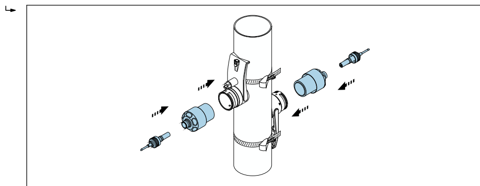
图 31 安装传感器并连接传感器电缆
