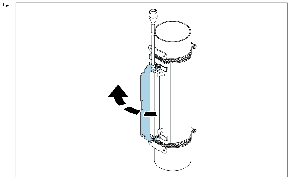
图 25 紧固传感器外壳
