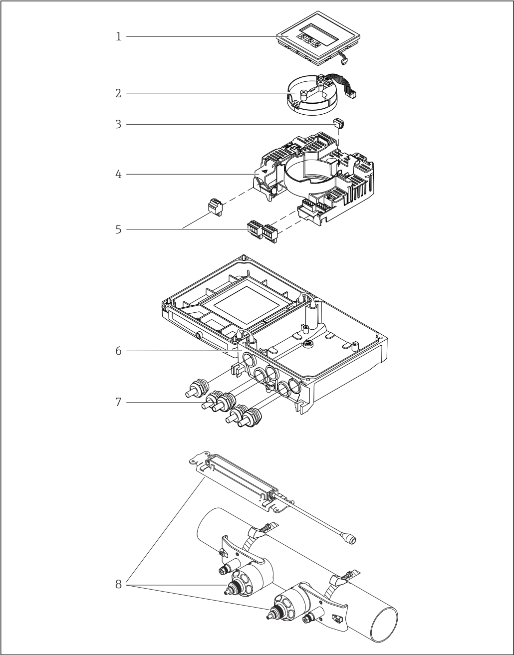
图 1 主要组成部件
