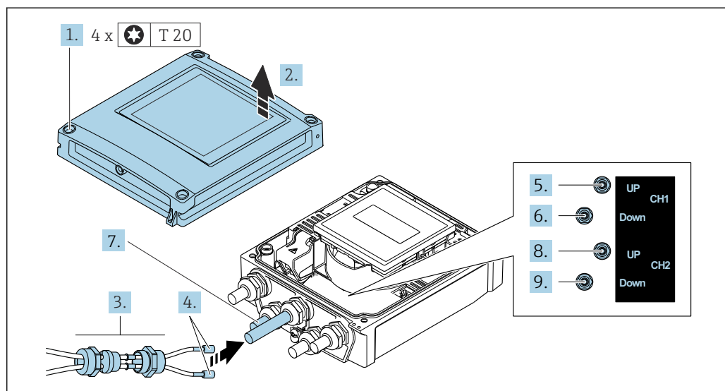
图 37 变送器：带接线端子的主要电子模块
