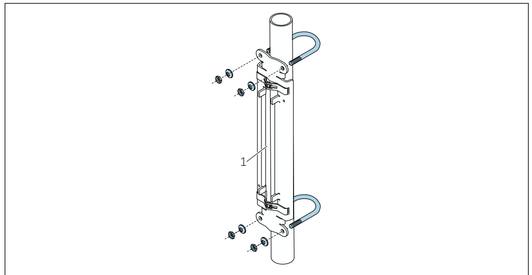
图 16 带 U 型螺丝的传感器安装支座
