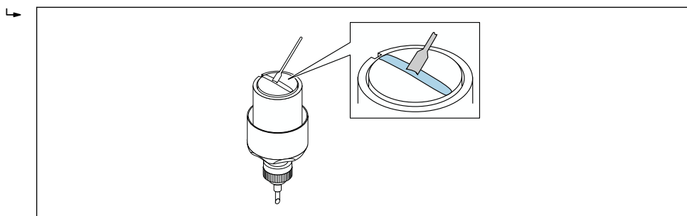
图 30 在传感器的接触面上涂抹耦合凝胶 (如果没有耦合垫)
