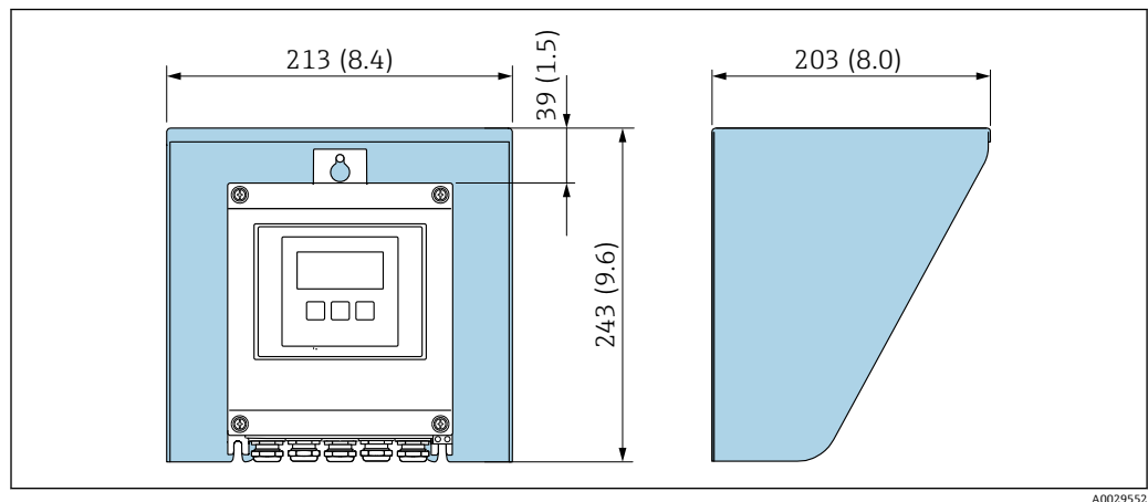
图 15 防护罩的外形尺寸示意图；单位：mm (in)
