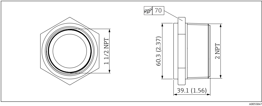
图 24 UNI 转接头的外形尺寸
