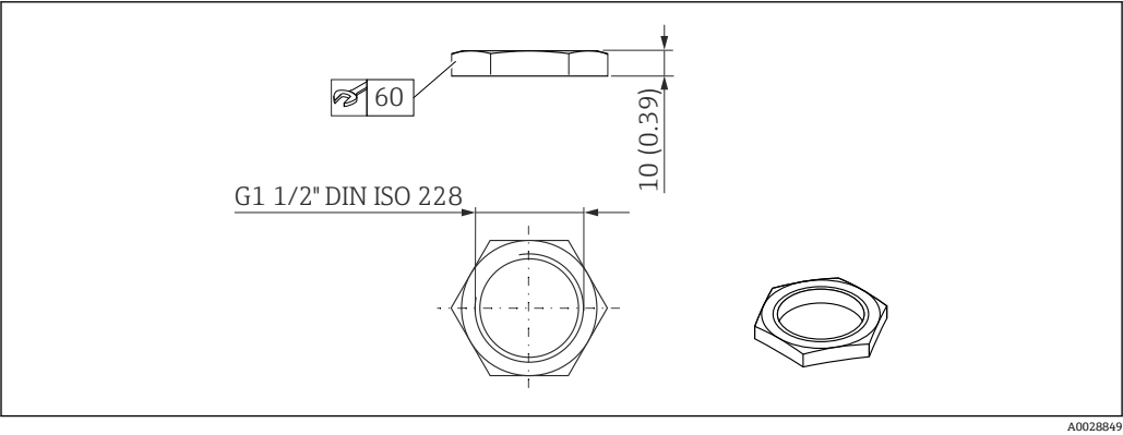
图 21 锁紧螺母的外形尺寸。测量单位 mm (in)
