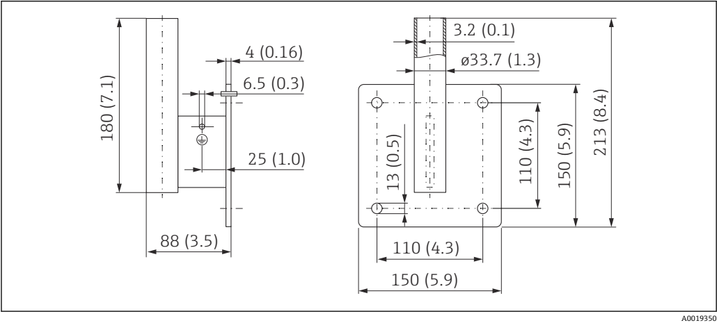
图 39 墙装架的外形尺寸。测量单位 mm (in)
