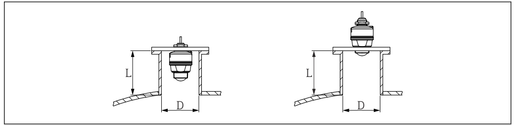
图 3 安装在安装短管中 (40 mm (1.5 in) 口径天线)
