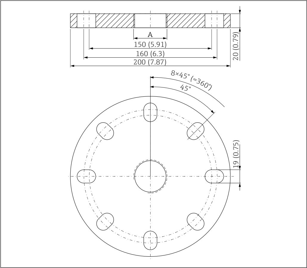
图 43 UNI 3"/DN80/80 法兰的外形尺寸示意图。测量单位 mm (in) A 传感器连接（产品选型表中的“天线端过程连接”或“电缆入口过程连接”）
