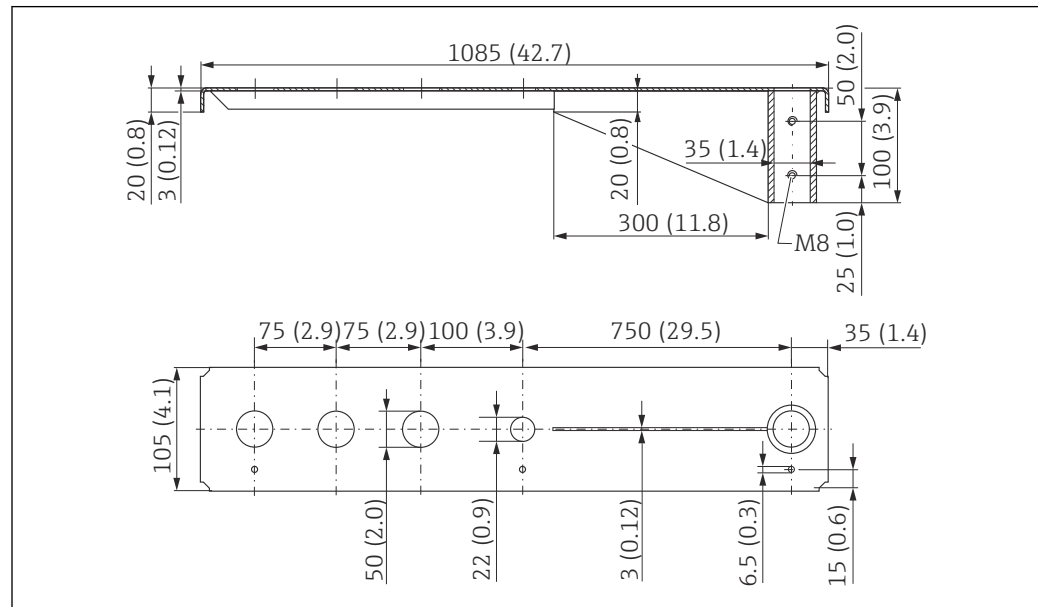
图 36 1000 mm 旋转悬臂的外形尺寸（安装在 G 1½" 传感器天线端过程连接上）。测量单位 mm (in)
