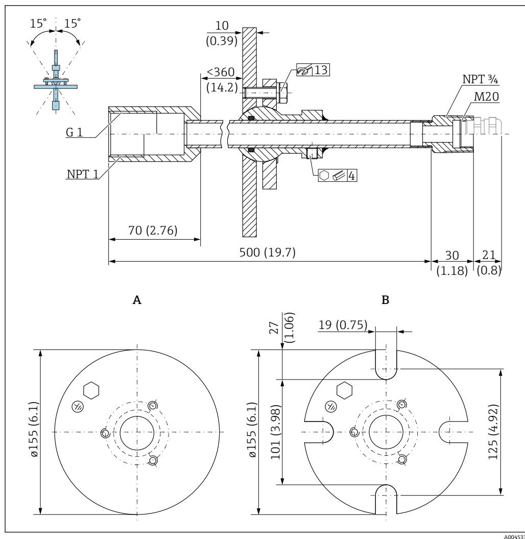
图 41 外形尺寸。测量单位 mm (in)
