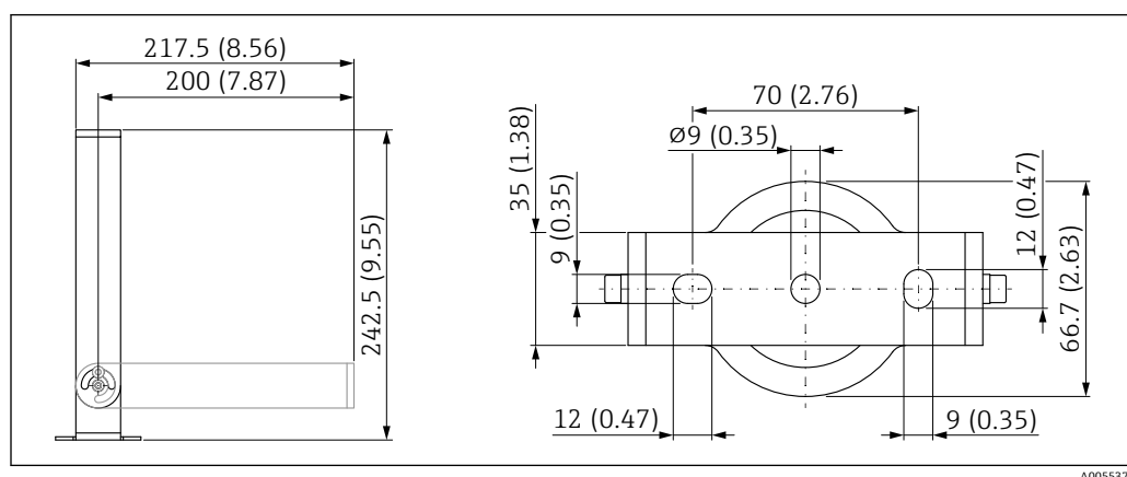
图 29 安装架的外形尺寸示意图。测量单位 mm (in)
