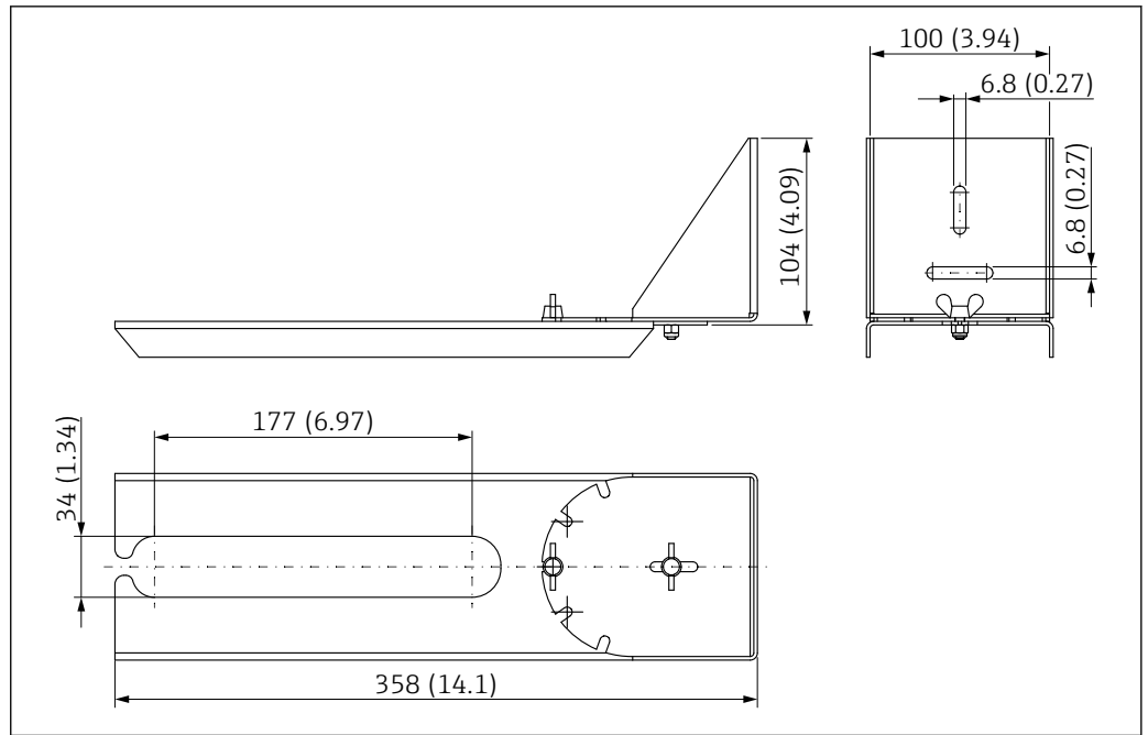
40 旋转安装架的外形尺寸。测量单位 mm (in)
