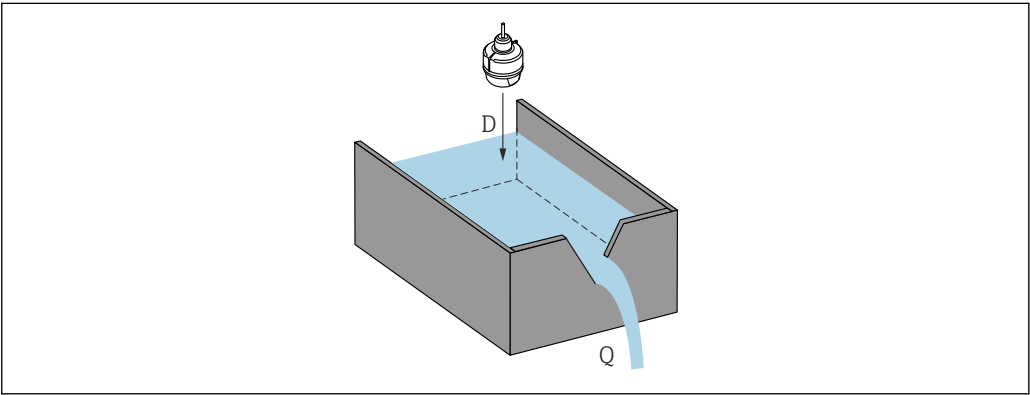
图 16 液体流量测量的设置参数
