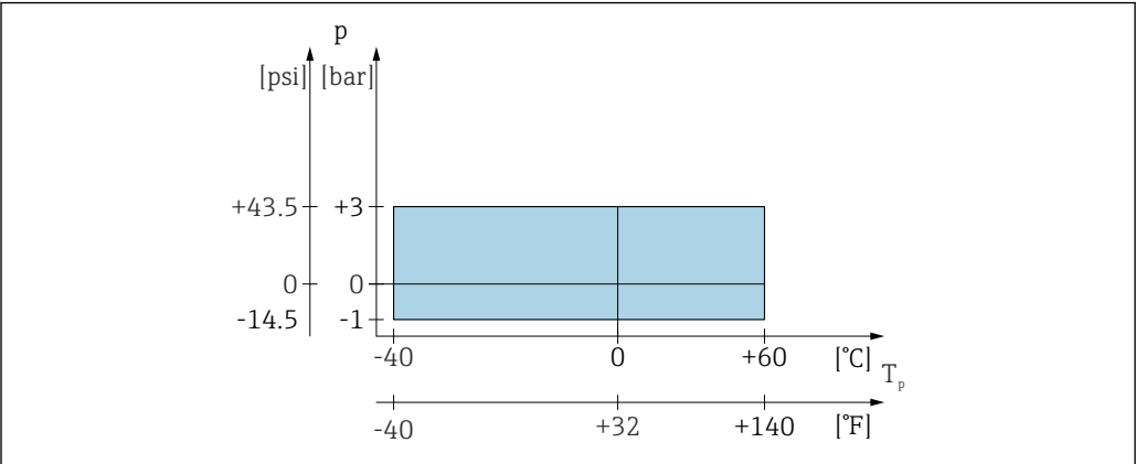
图 46 允许过程温度和过程压力
