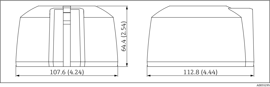
图 20 G1/NPT1 防护罩的外形尺寸（顶部电缆入口）。测量单位 mm (in)
