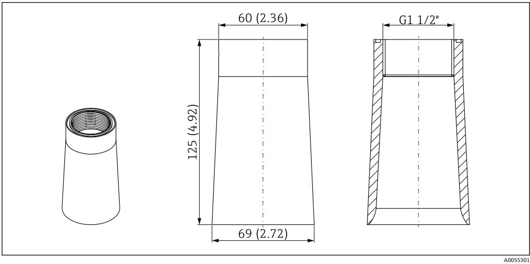
图 25 40 mm (1.5 in)防溢管的外形尺寸。测量单位 mm (in)
