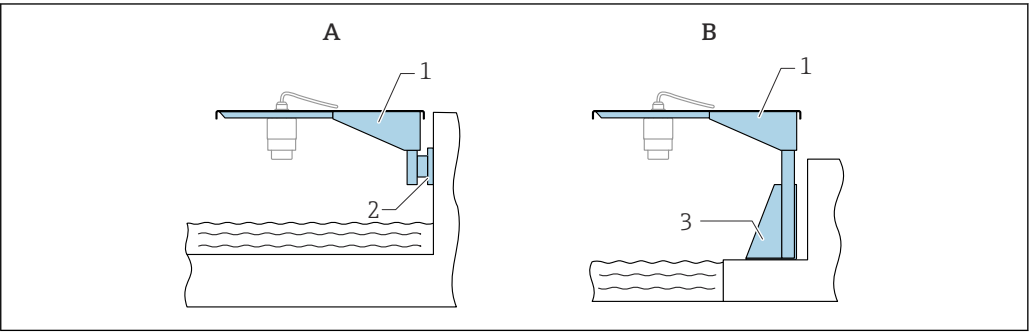
图 31 传感器电缆入口过程连接的安装方式
