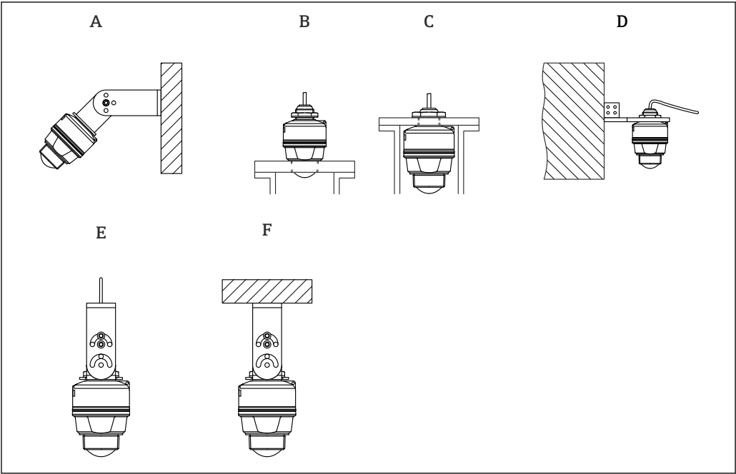
图 2 安装在墙壁或罐顶上
