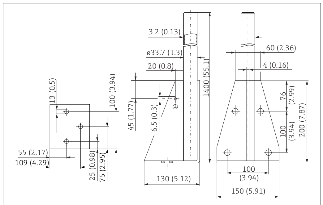
图 38 外形尺寸。测量单位 mm (in)
