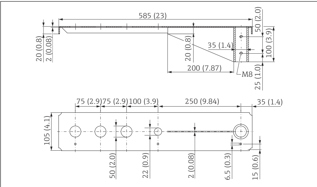
图 35 500 mm 旋转悬臂的外形尺寸（安装在 G 1½"传感器天线端过程连接上）。测量单位 mm (in)
