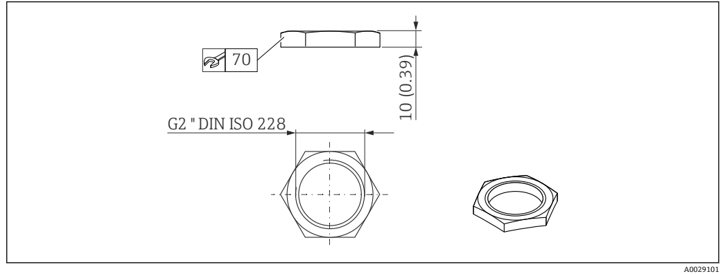
图 22 锁紧螺母的外形尺寸。测量单位 mm (in)
