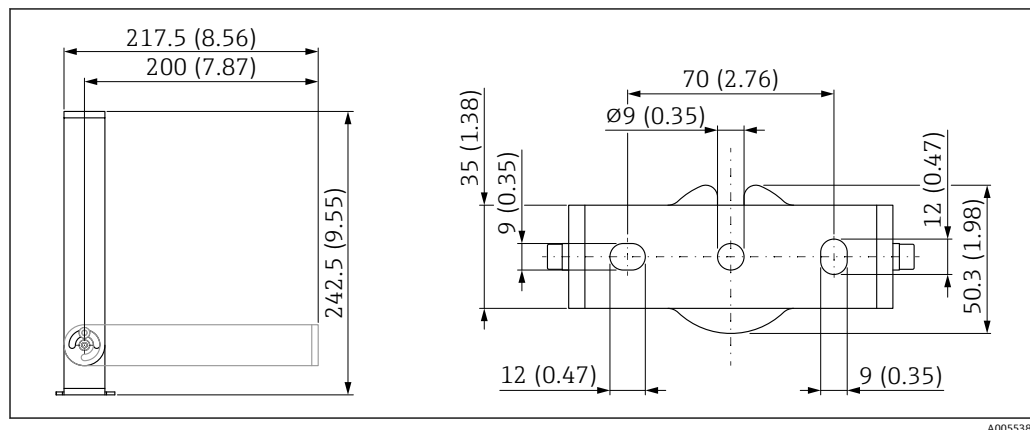
图 28 安装架的外形尺寸示意图。测量单位 mm (in)
