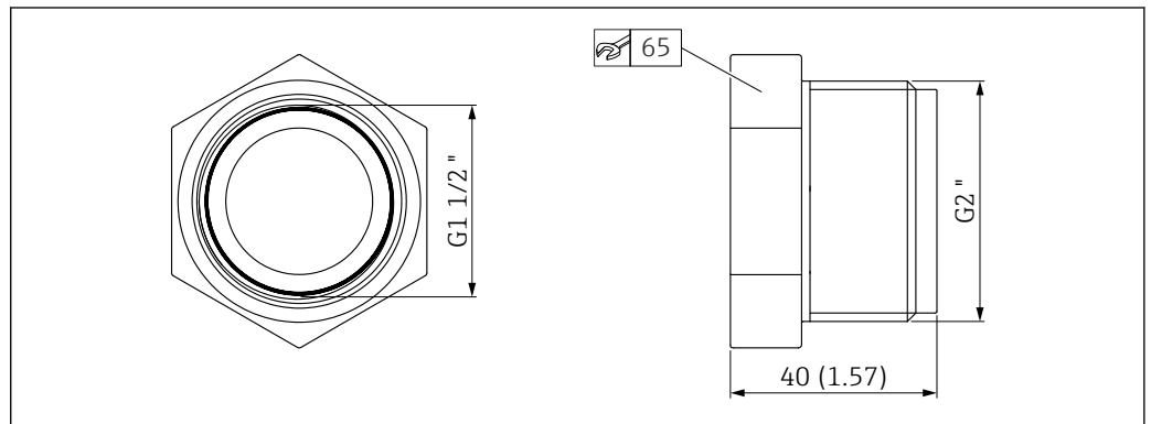
图 23 UNI 转接头的外形尺寸
