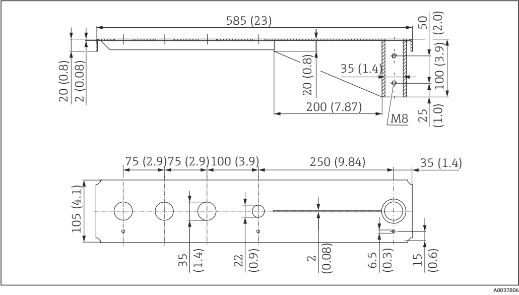
32 500 mm 旋转悬臂的外形尺寸（安装在传感器电缆入口过程连接上）。测量单位 mm (in)
