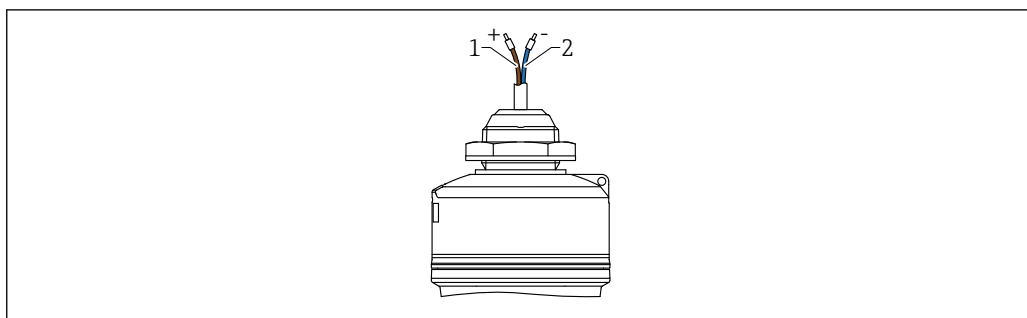
图 10 电缆分配，从上方接入电缆
