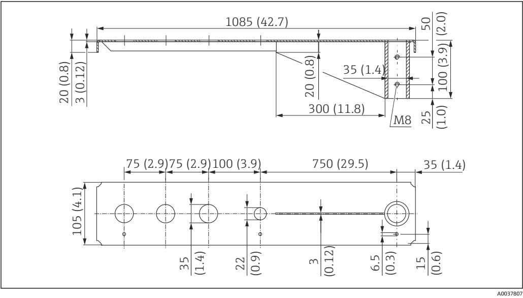
33 1000 mm 旋转悬臂的外形尺寸（安装在传感器电缆入口过程连接上）。测量单位 mm (in)
