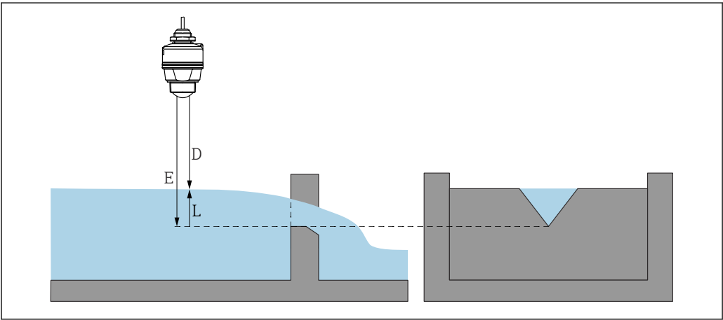
图 18 实例：三角堰
