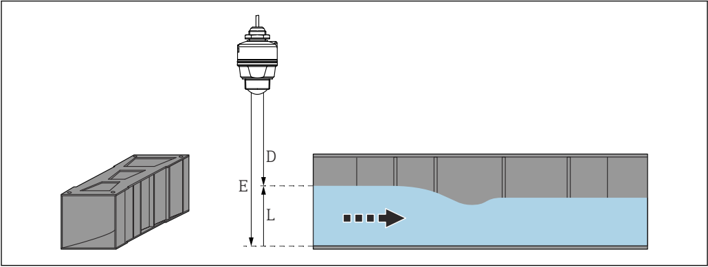
图 17 实例：文丘里水槽
