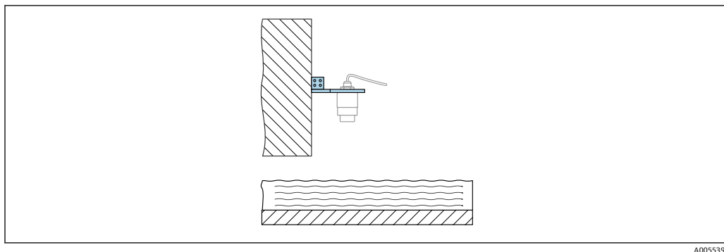
图 9 使用悬臂和墙装架安装，悬臂可以旋转和调节（例如在水渠正上方定位设备）
