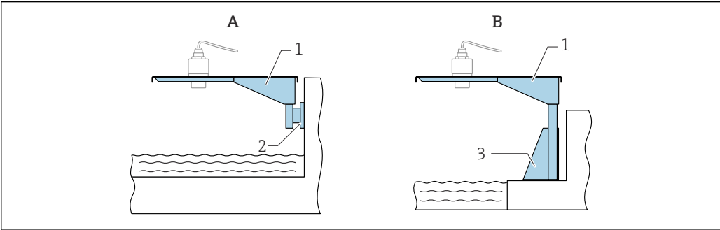
图 34 传感器天线端过程连接的安装方式
