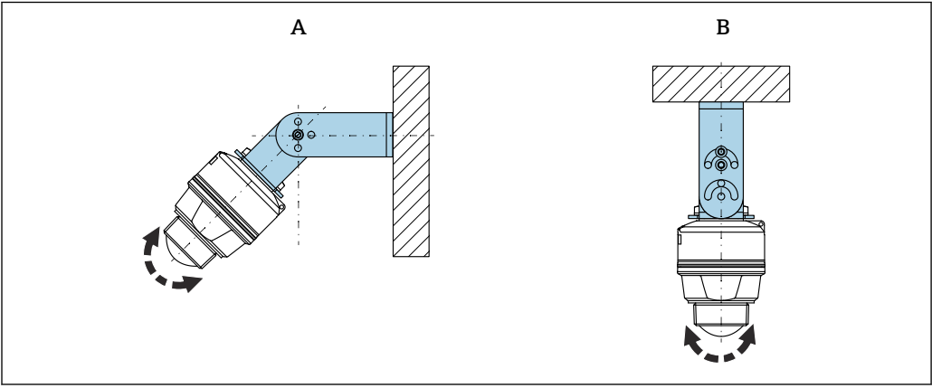
图 6 使用安装架安装（可调节）
