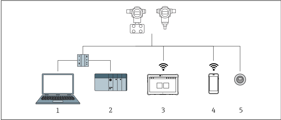
☐ 12 PROFINET 프로토콜을 통한 원격 작동 옵션
