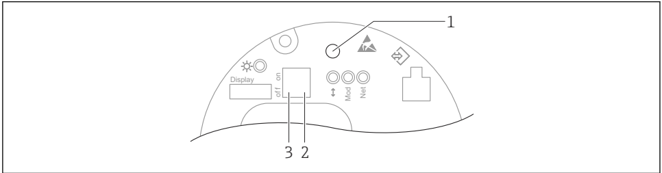
☒ 6 Ethernet-APL 전자 부속품의 작동 키 및 DIP 스위치
