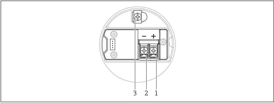
5 연결부의 연결 단자 및 접지 단자
