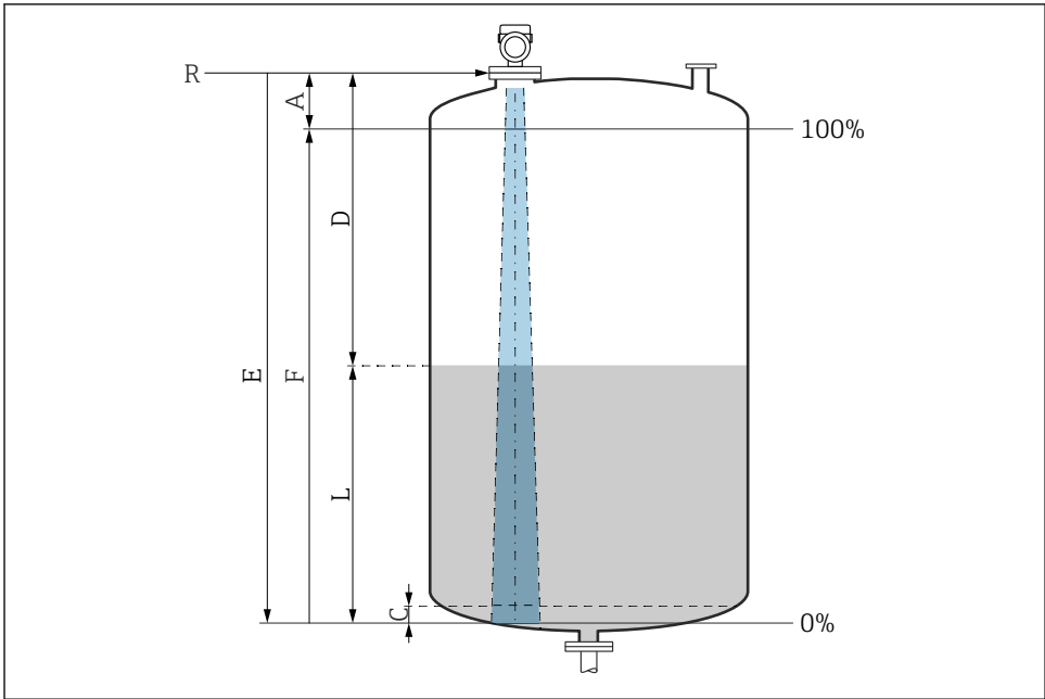
13 액체 레벨 측정 구성 파라미터
