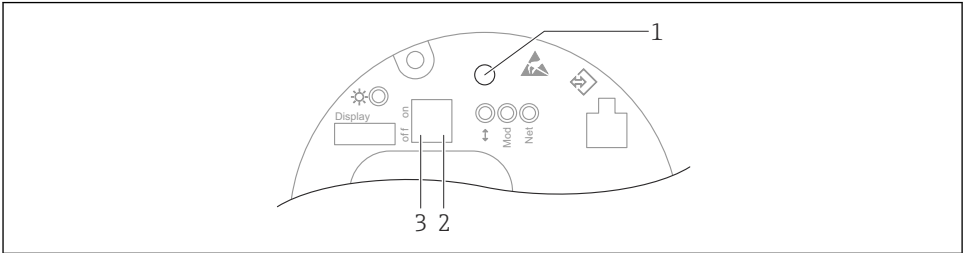
图 6 Ethernet-APL 电子插件上的操作按键和 DIP 开关
