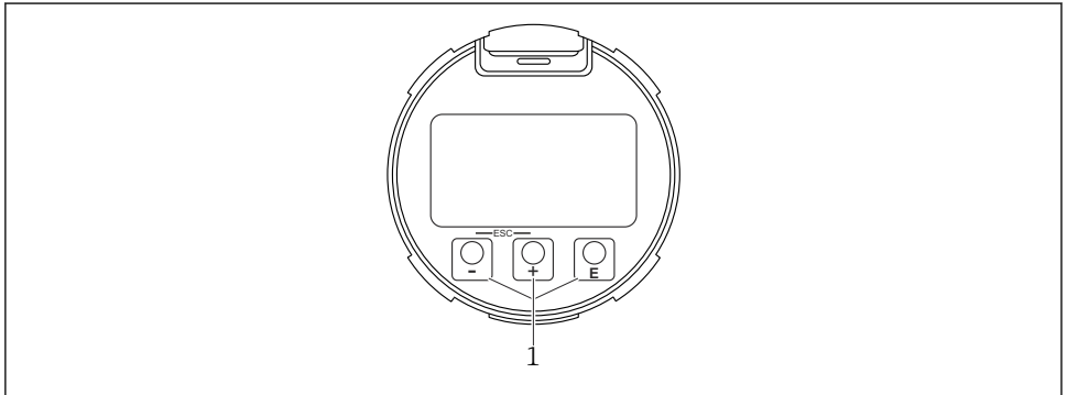
图 7 图形显示屏，带光敏按钮 (1)
