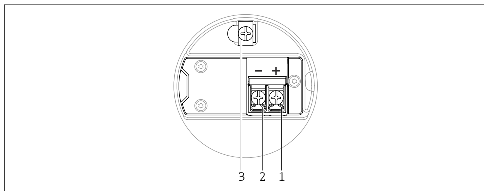
図 7 端子部の接続端子と接地端子
