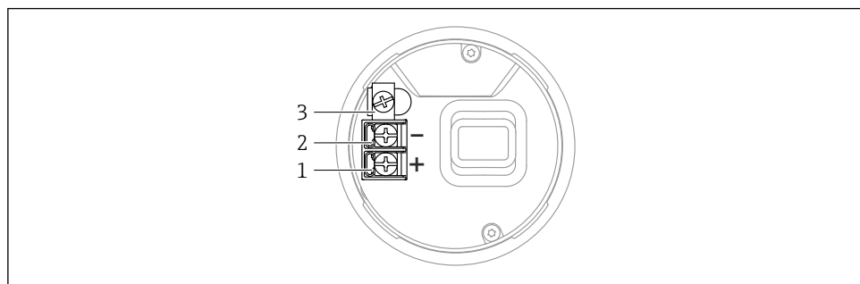
図 6 端子部の接続端子と接地端子（シングルコンパートメントハウジング）
