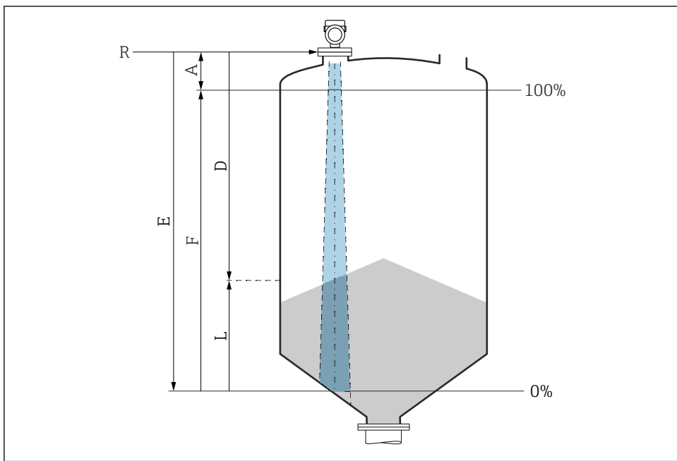
図 16 粉体のレベル測定用パラメータの設定
