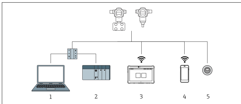
図 15 PROFINET プロトコル経由のリモート操作用オプション
