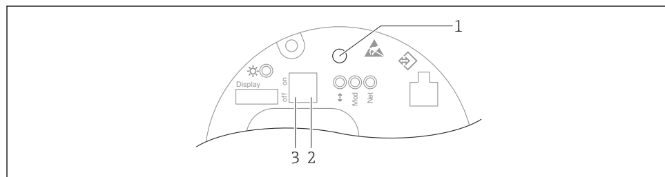
図 9 Ethernet-APL エレクトロニックインサート上の操作キーおよび DIP スイッチ
