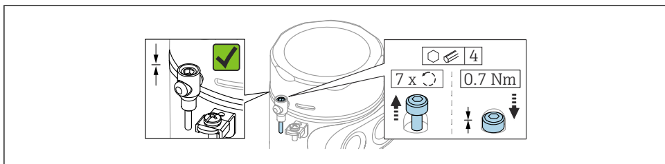
図 5 固定ねじ付きカバー；サニタリハウジング（粉塵防爆仕様のみ）
