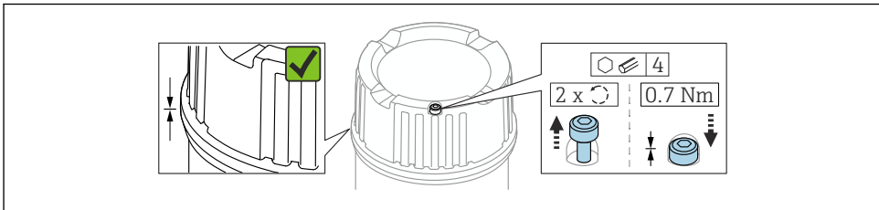
図 4 固定ねじ付きカバー
